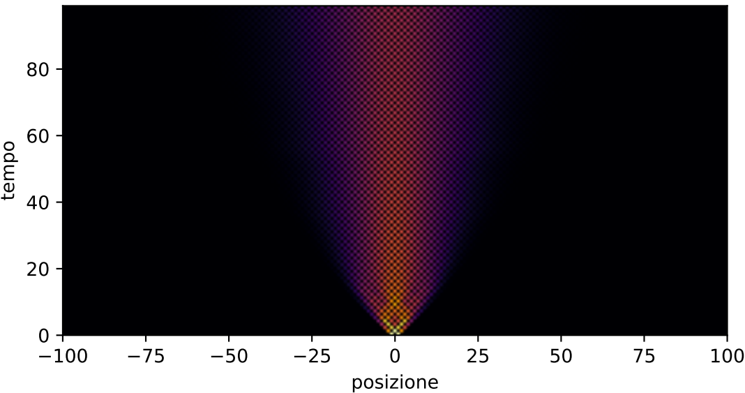
Passeggiata aleatoria quantistica, canale meas, p=0.59
