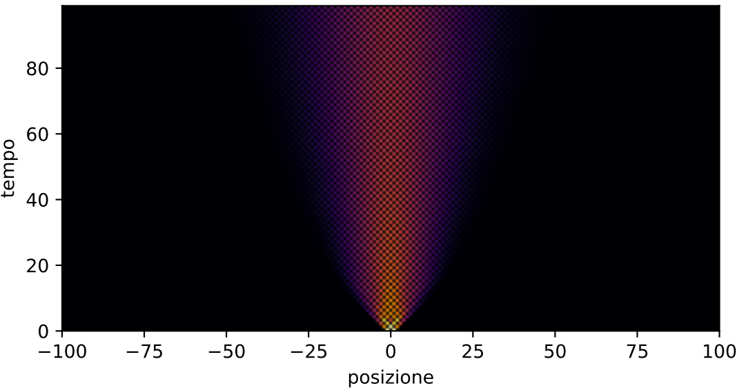
Passeggiata aleatoria quantistica, canale meas, p=0.67
