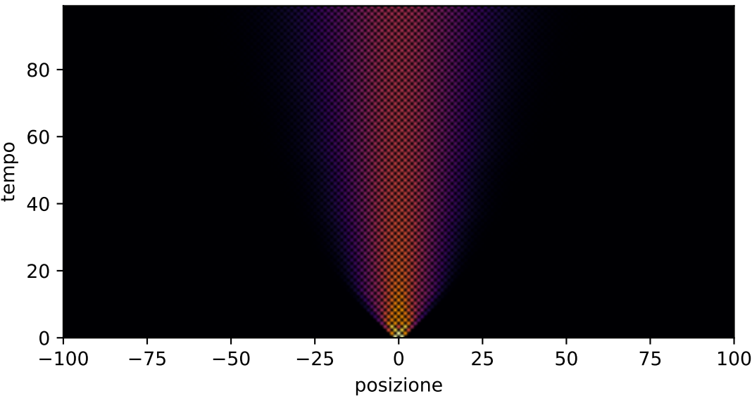
Passeggiata aleatoria quantistica, canale meas, p=0.69
