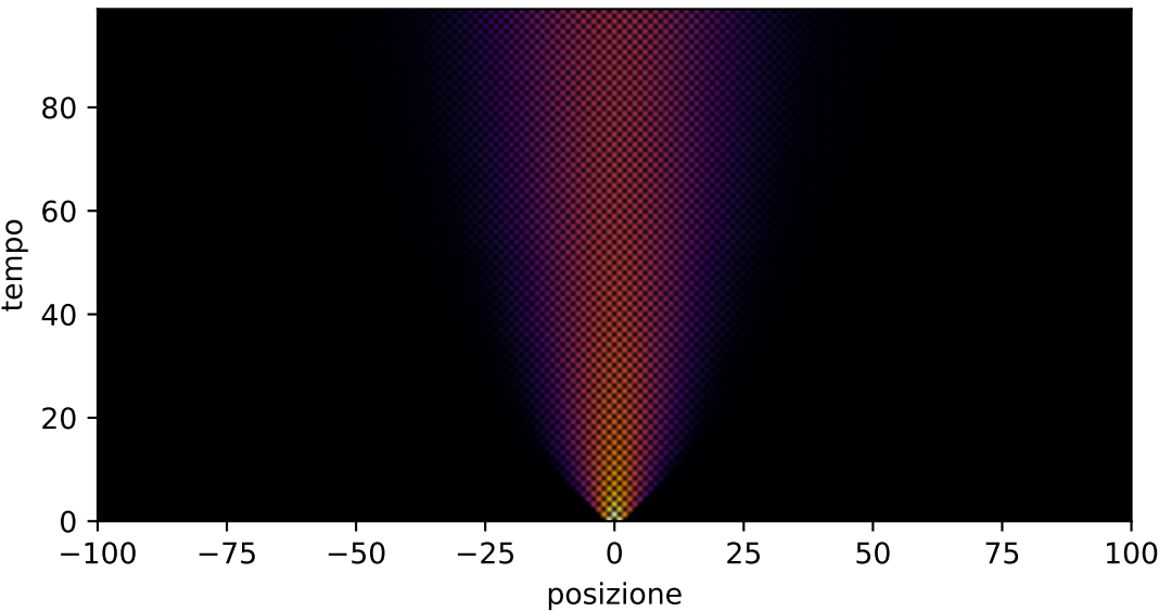
Passaggiata aleatoria quantistica, canale meas, p=0.74
