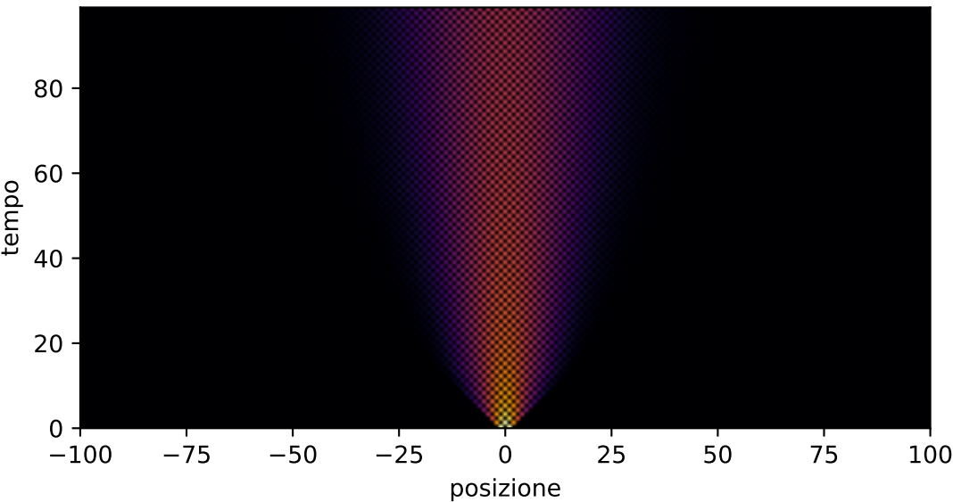
Passeggiata aleatoria quantistica, canale meas, p=0.82
