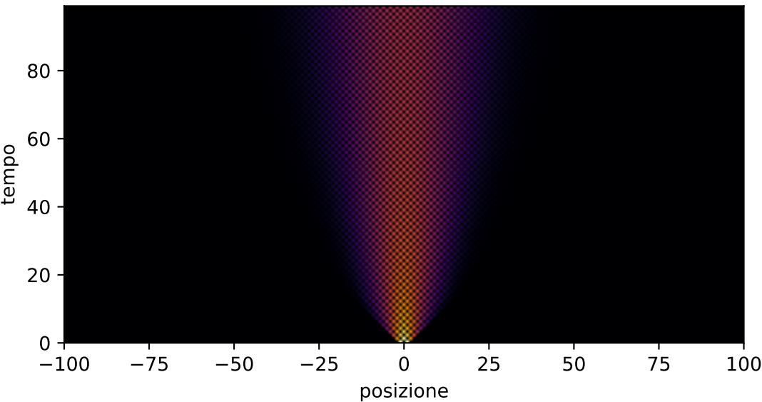
Passaggiata aleatoria quantistica, canale meas, p=0.85
