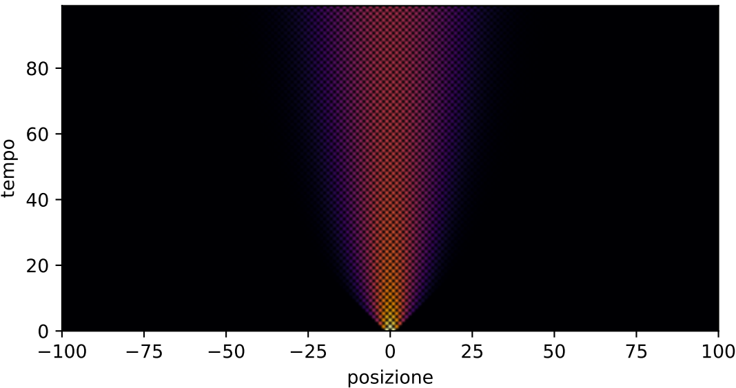
Passeggiata aleatoria quantistica, canale meas, p=0.95
