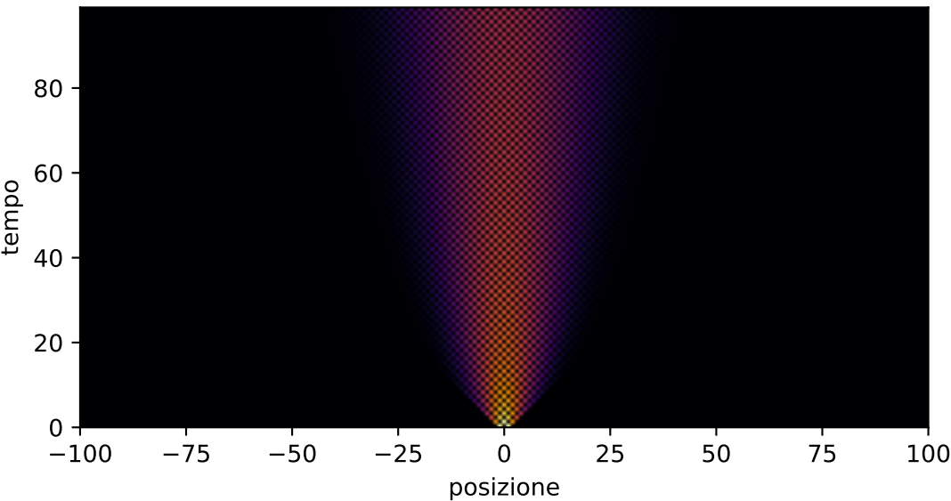
Passeggiata aleatoria quantistica, canale meas, p=1.0
