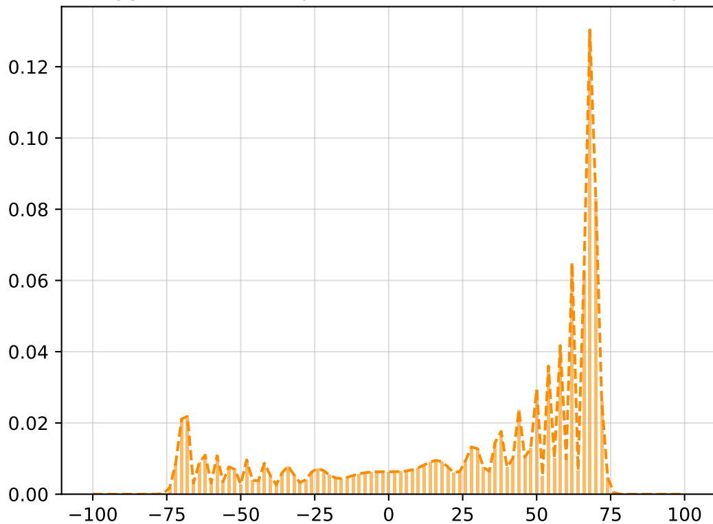
Passeggiata aleatoria quantistica senza correzione, 100 passi
