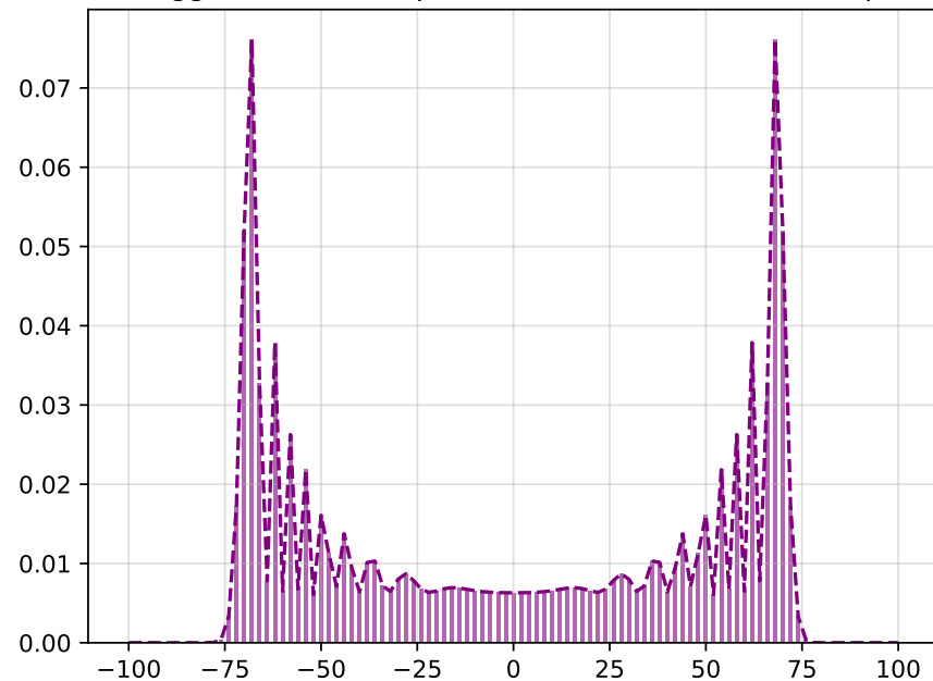
Passeggiata aleatoria quantistica con correzione, 100 passi
