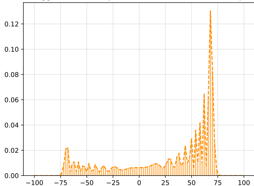
Passeggiata aleatoria quantistica senza correzione, 100 passi
