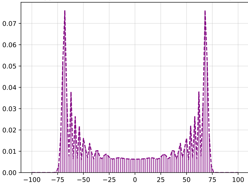
Passeggiata aleatoria quantistica con correzione, 100 passi
