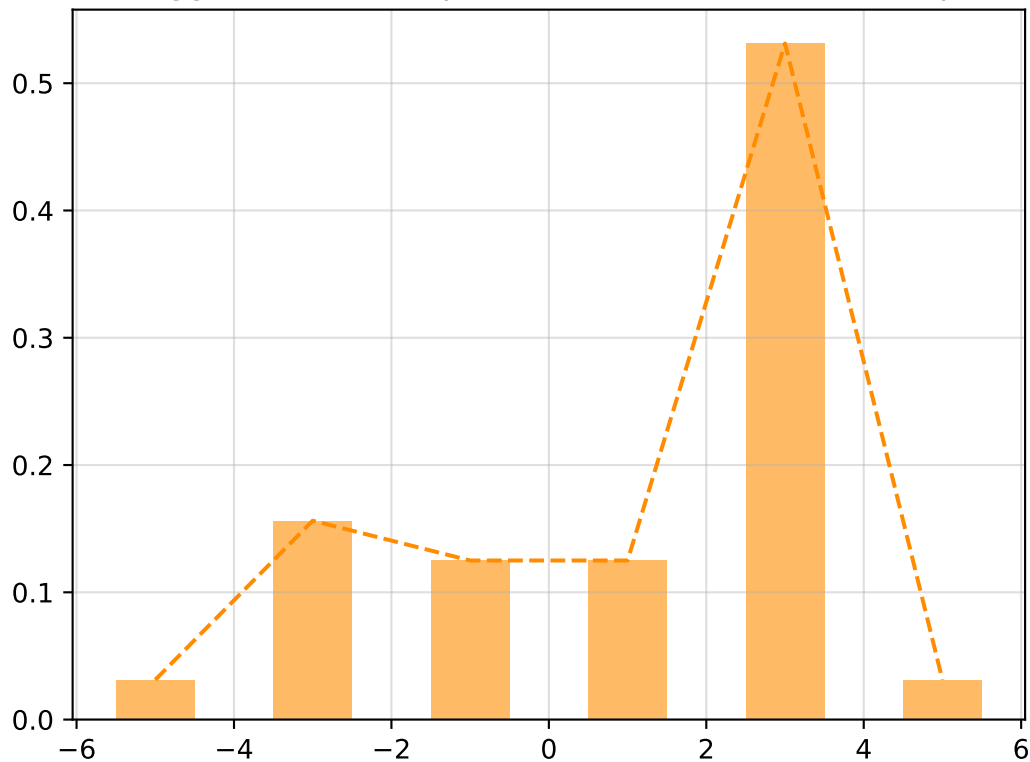
Passeggiata aleatoria quantistica senza correzione, 5 passi
