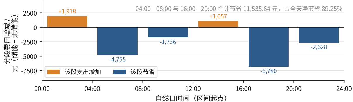
e 储能相对无储能的4小时分段费用增减
