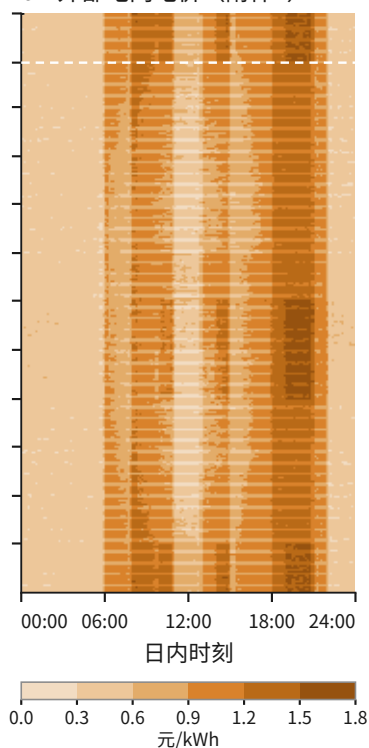
c 外部电网电价 (附件4)
