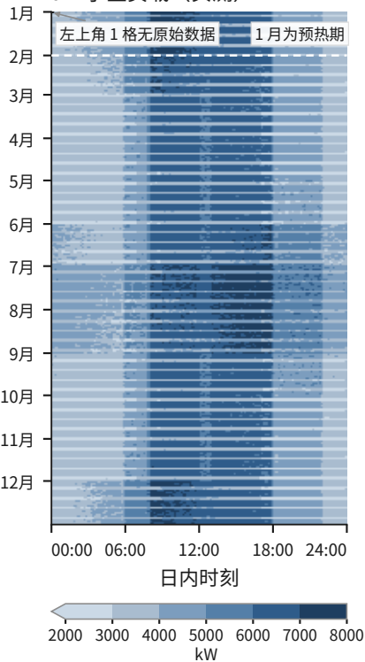
a 小区负载 (实测)
