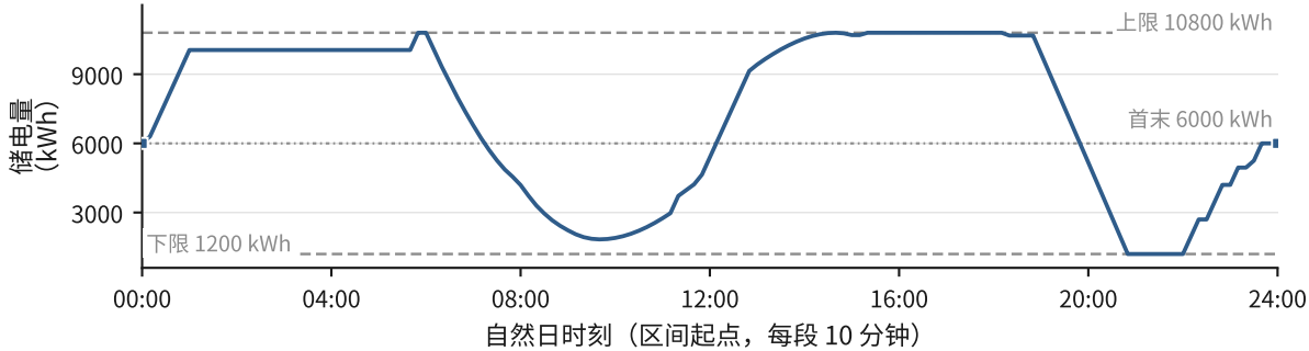
c 储电量轨迹与容量边界（方块为起止锚点）
