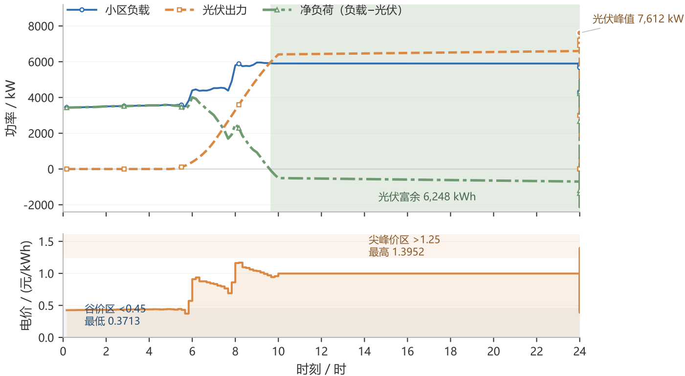
典型日（附件1）功率曲线与分时电价
