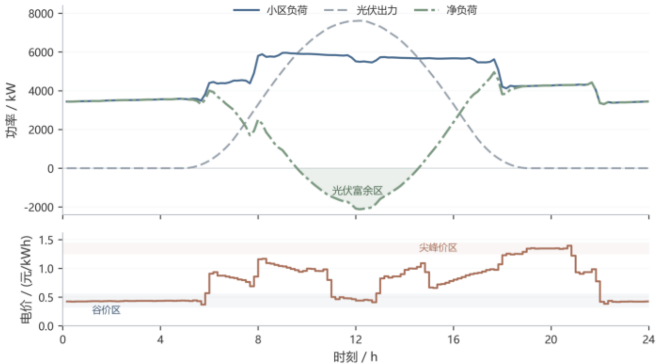
图 1b 典型日负荷、光伏、净负荷与分时电价
