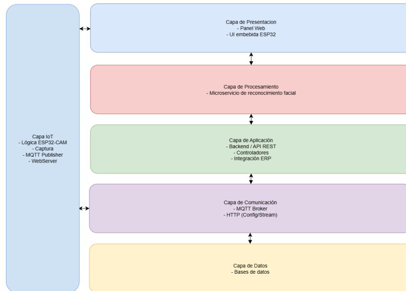
Figura 4.2: Arquitectura lógica
