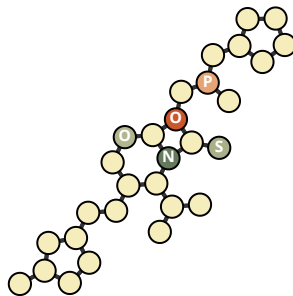
Cefazolin Sodium
