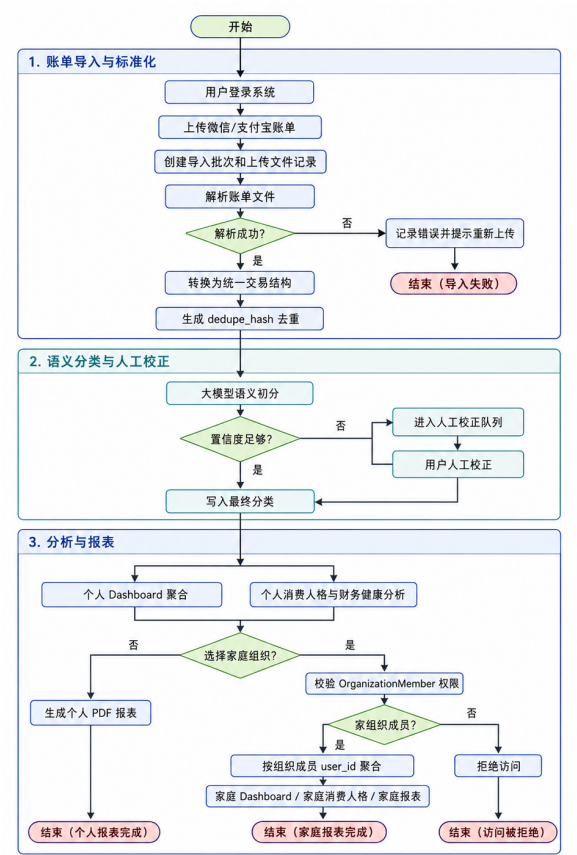
图 3.2 核心业务活动图
