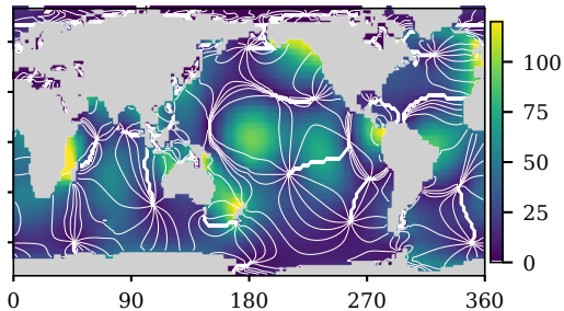
(d) NN-8 M_2 amplitude [cm], phase every 30^\circ
