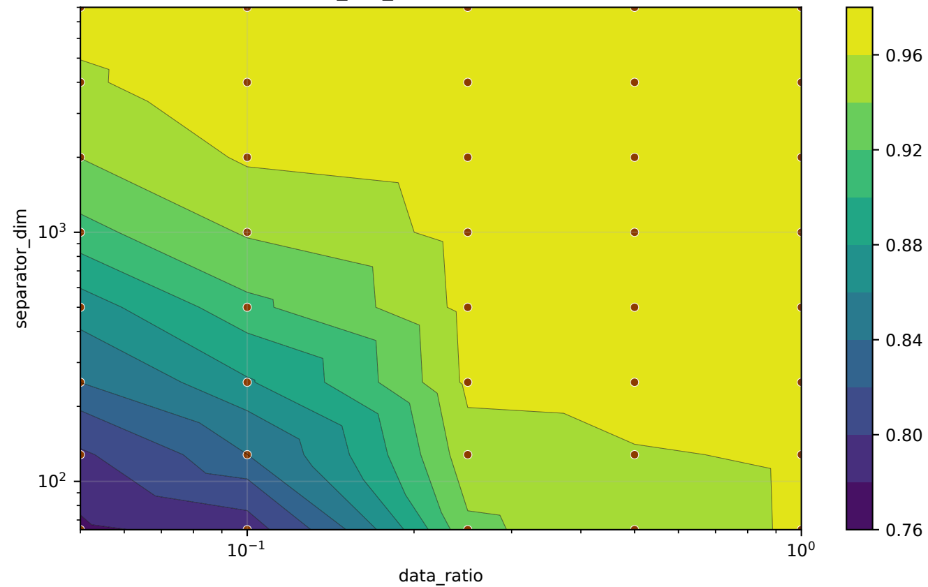
val/align_cka_hidden (steps=all, last)
