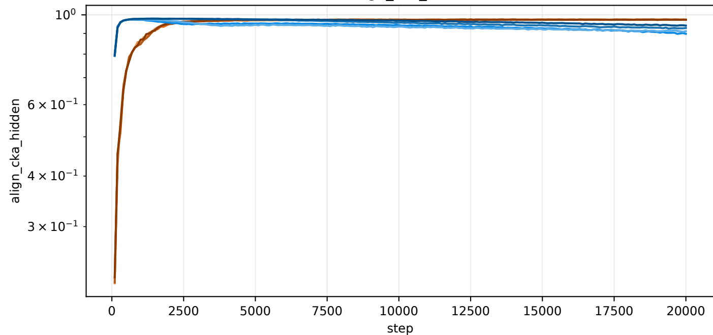
val/align_cka_hidden
