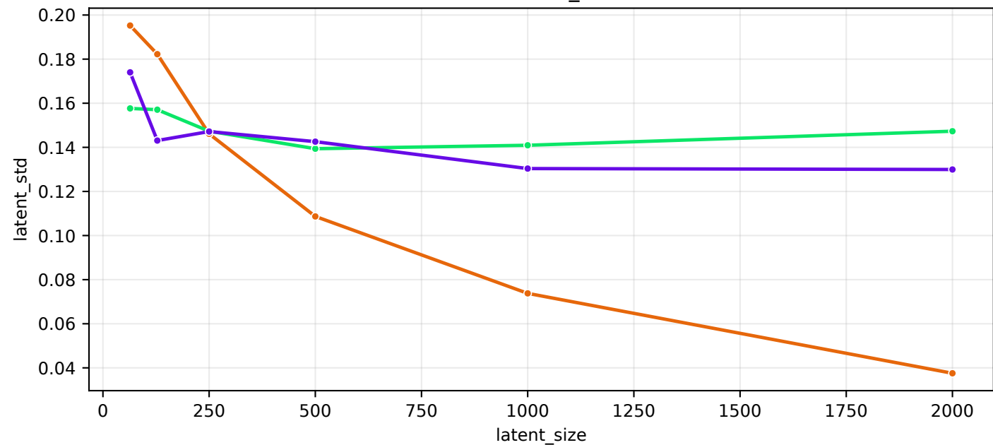
val/latent_std
