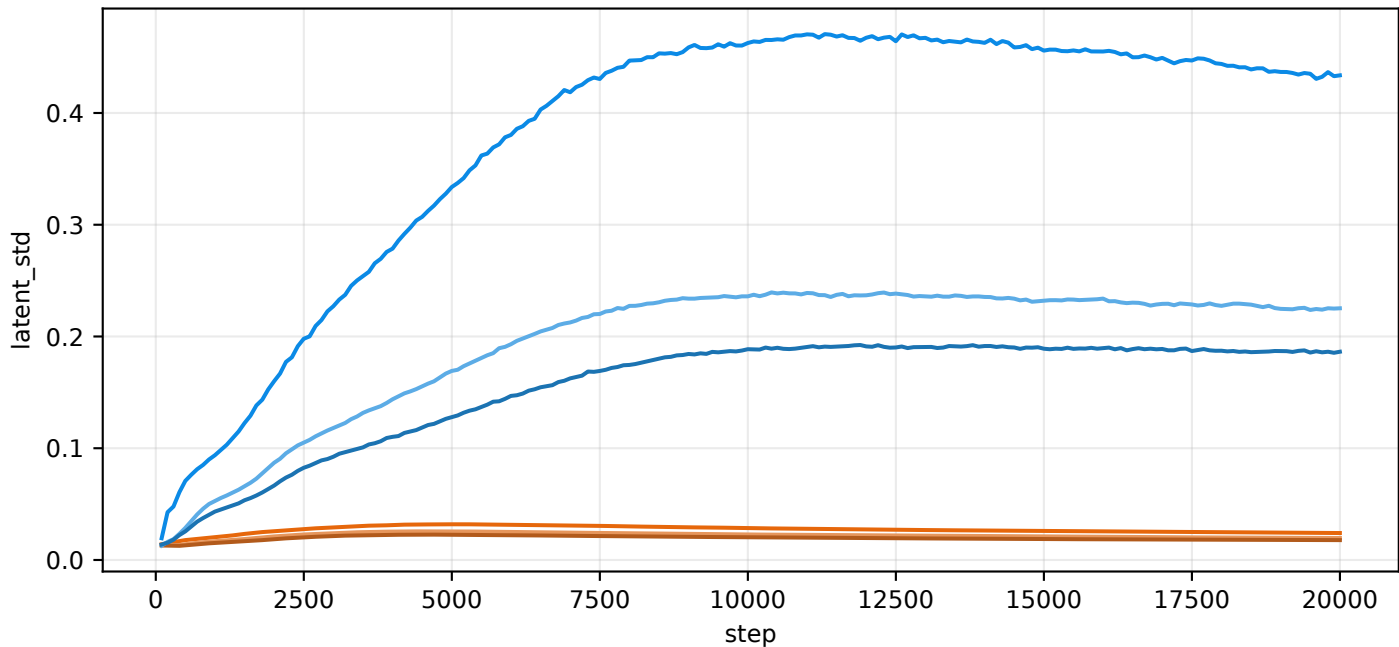
val/latent_std
