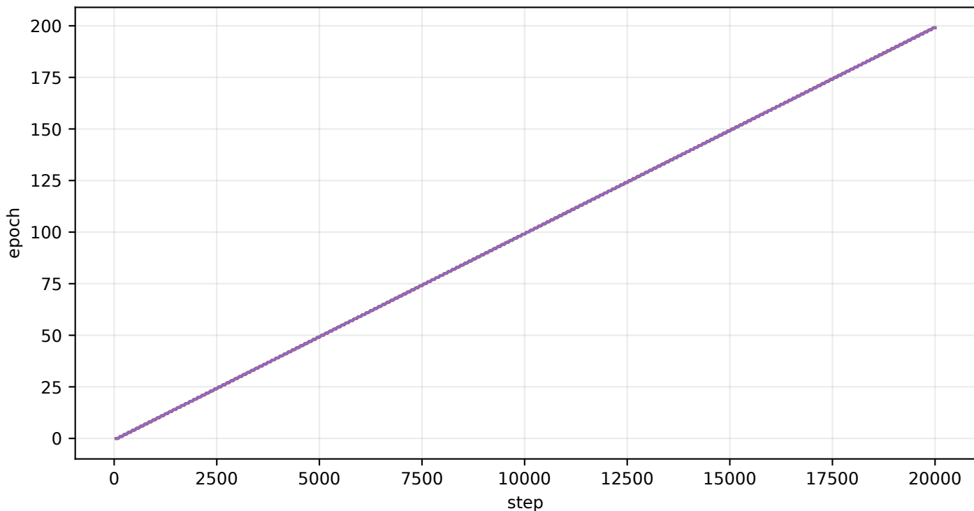
epoch
