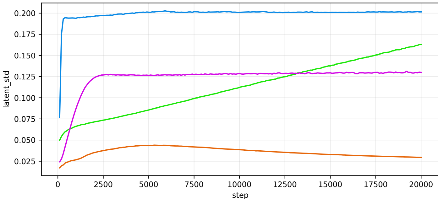
val/latent_std
