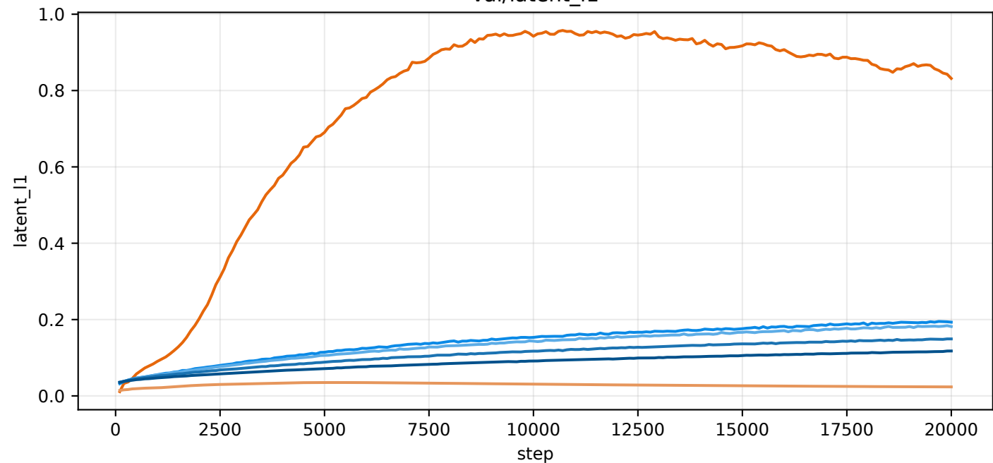
val/latent_l1
