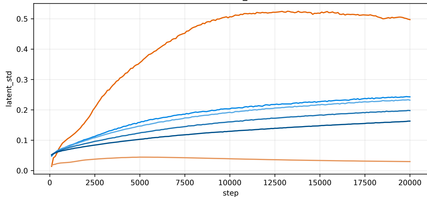
val/latent_std
