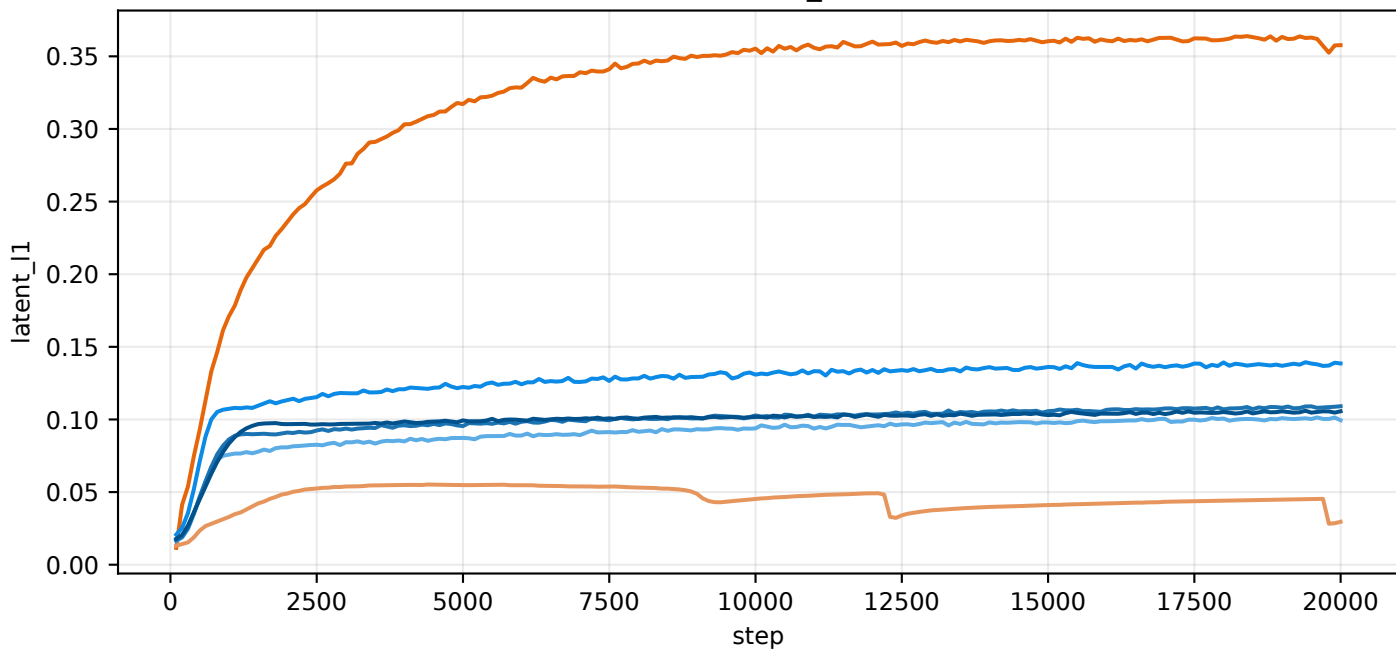
val/latent_l1
