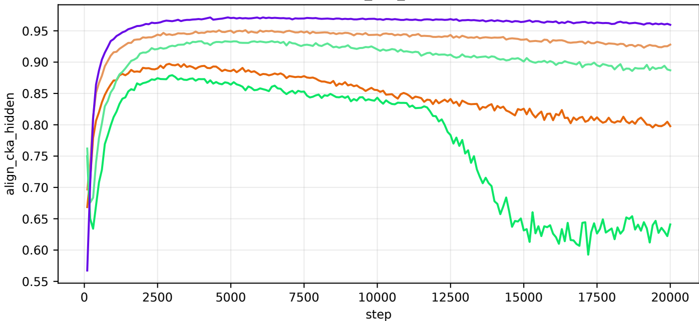
val/align_cka_hidden
