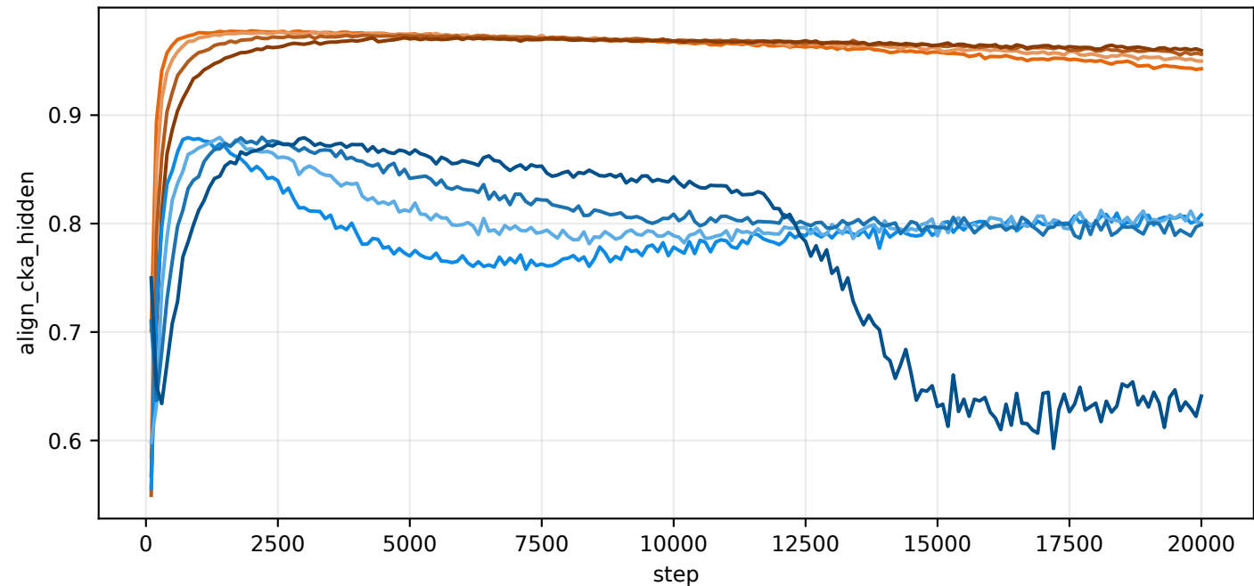
val/align_cka_hidden
