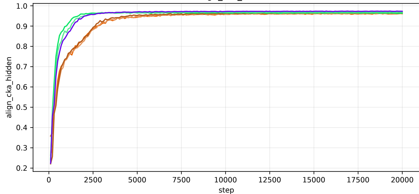
val/align_cka_hidden
