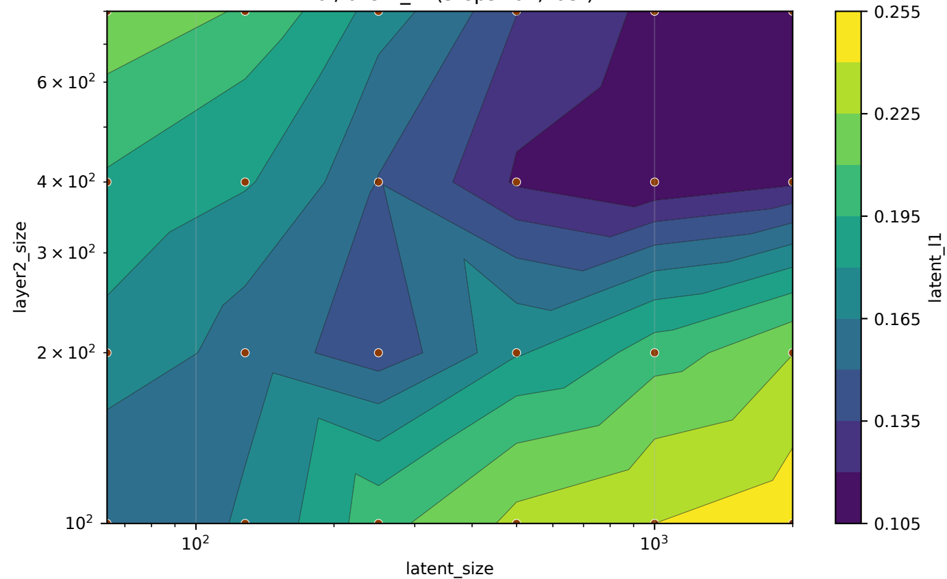
val/latent_l1 (steps=all, last)
