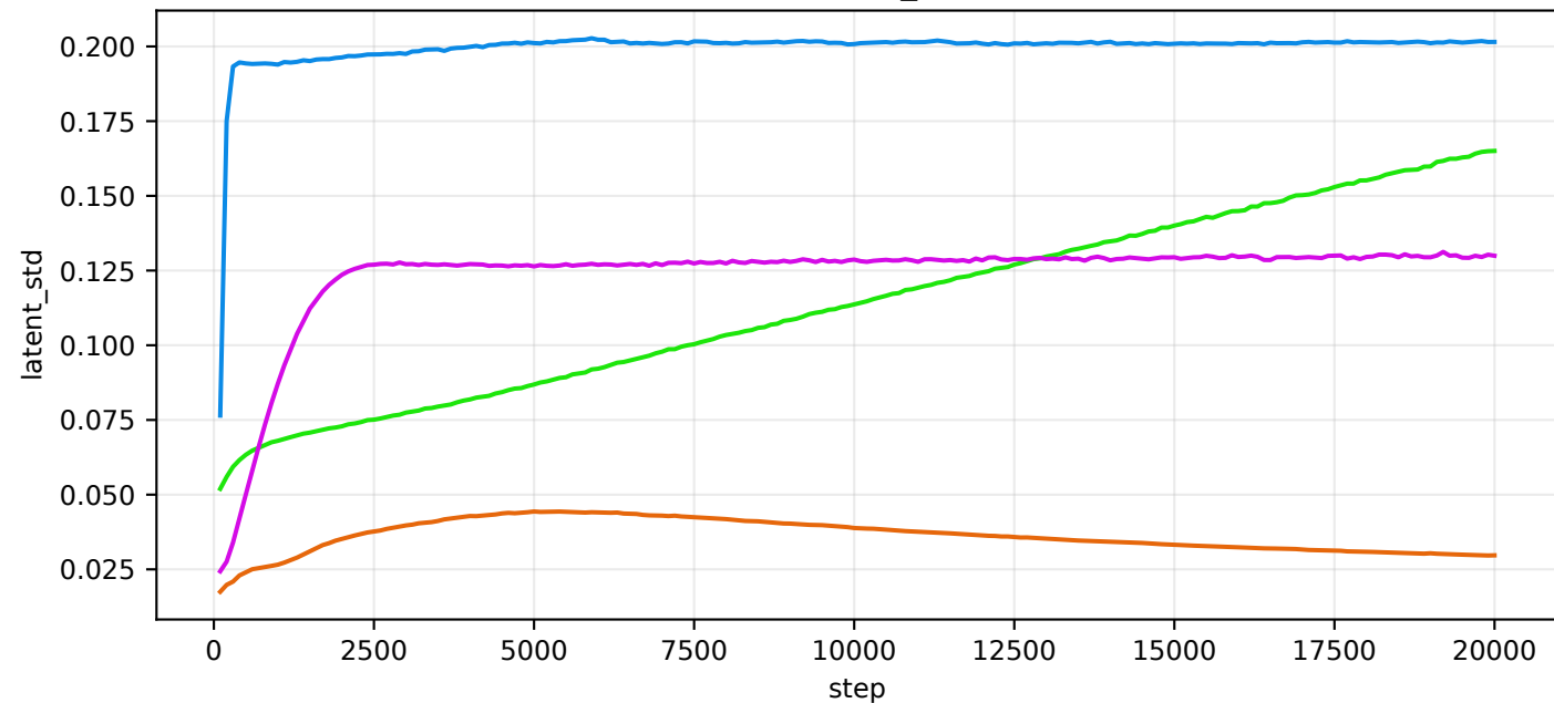
val/latent_std
