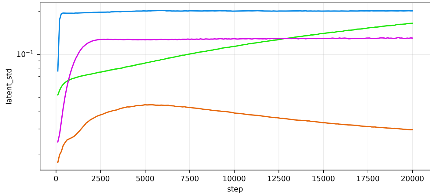
val/latent_std
