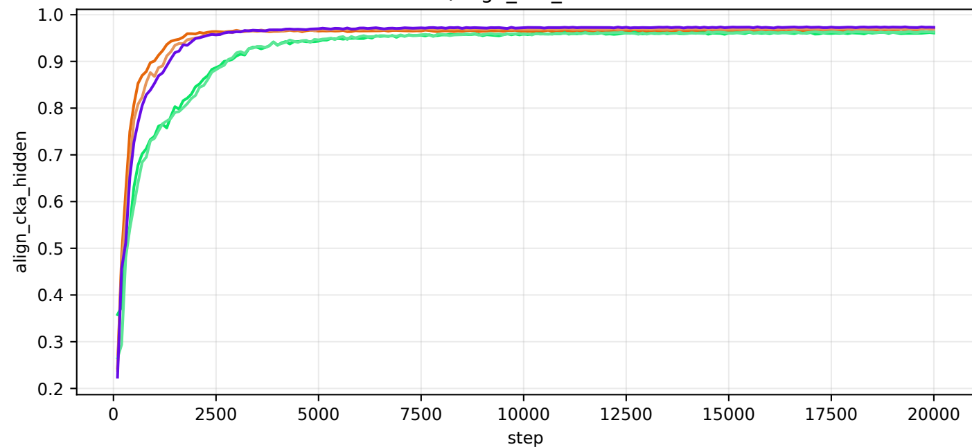
val/align_cka_hidden
