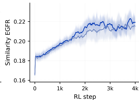
Similarity EGFR
