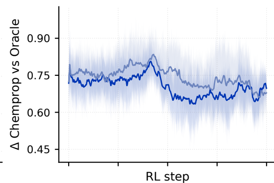
Similarity EGFR
