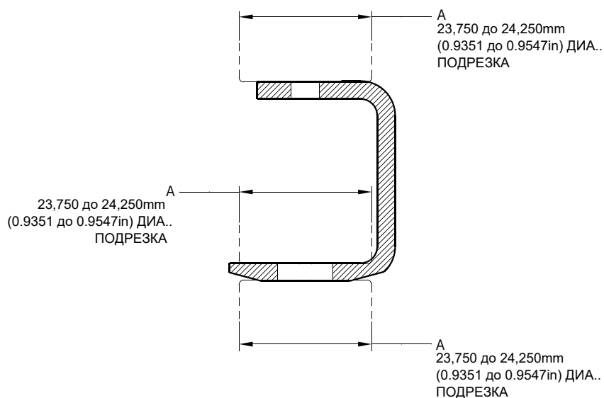
СЕЧЕНИЕ Z-Z
