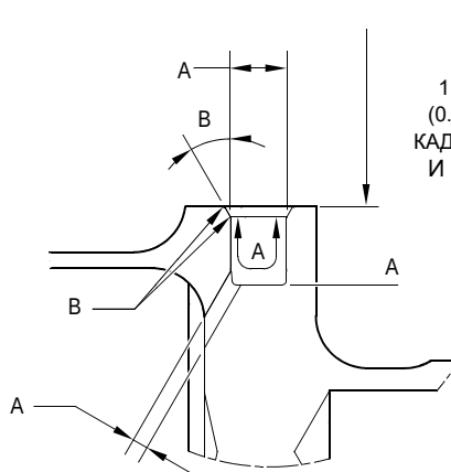
ДЕТАЛЬ Y
