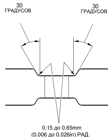
ДЕТАЛЬ E
