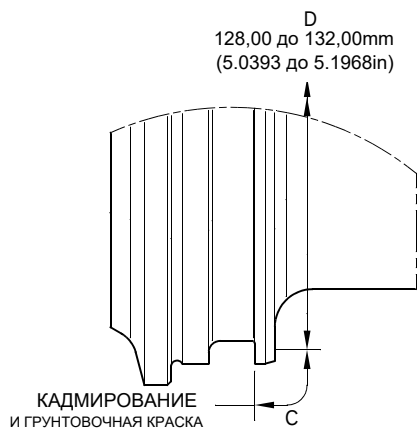
ДЕТАЛЬ X
