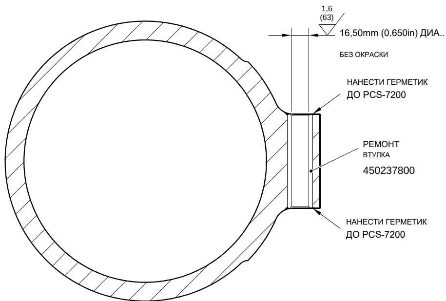
СЕЧЕНИЕ Z-Z
