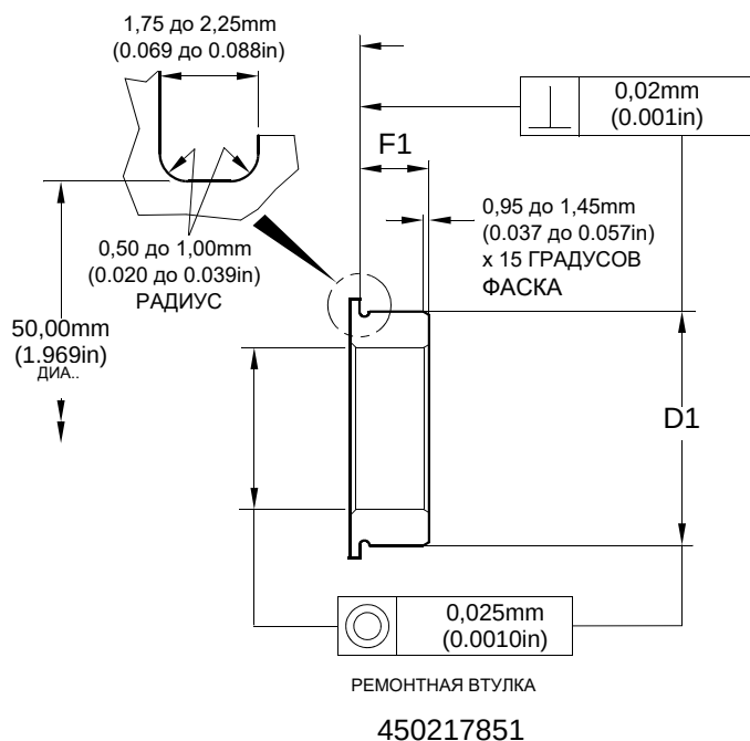
Ремонт корпуса стойки – мехобработка Рисунок 602
