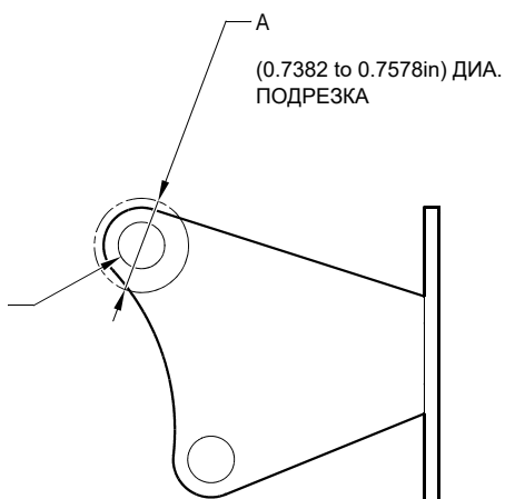
ВИД А
