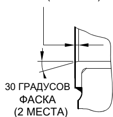
ДЕТАЛЬ X
