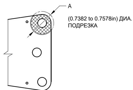
ВИД С
