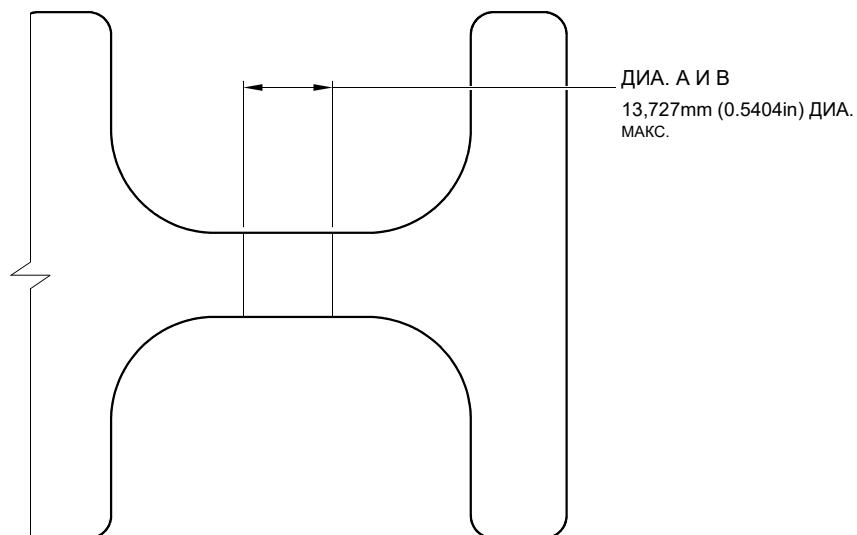
СЕЧЕНИЕ Y-Y (БЕЗ ВТУЛОК)
