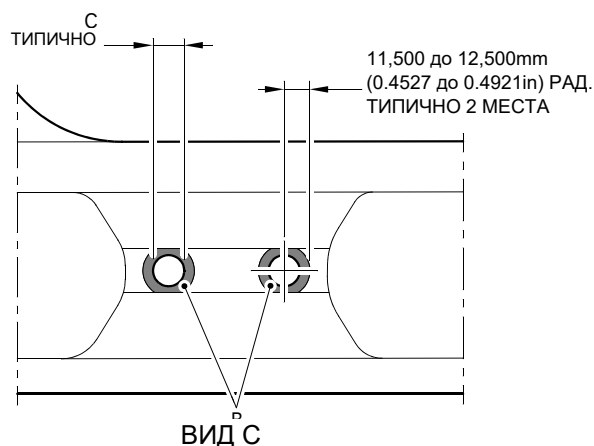
ВИД С ДЛЯ КОРПУСА СТОЙКИ (20-410В, 20-420В, 20-410D И 20-420D) ТОЛЬКО
