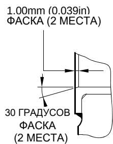
ДЕТАЛЬ X
