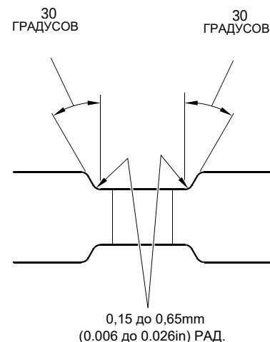
ДЕТАЛЬ Е
