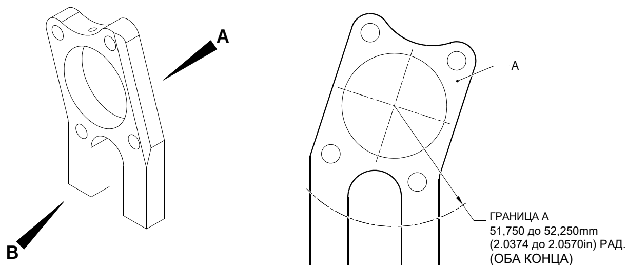
ВИД А
