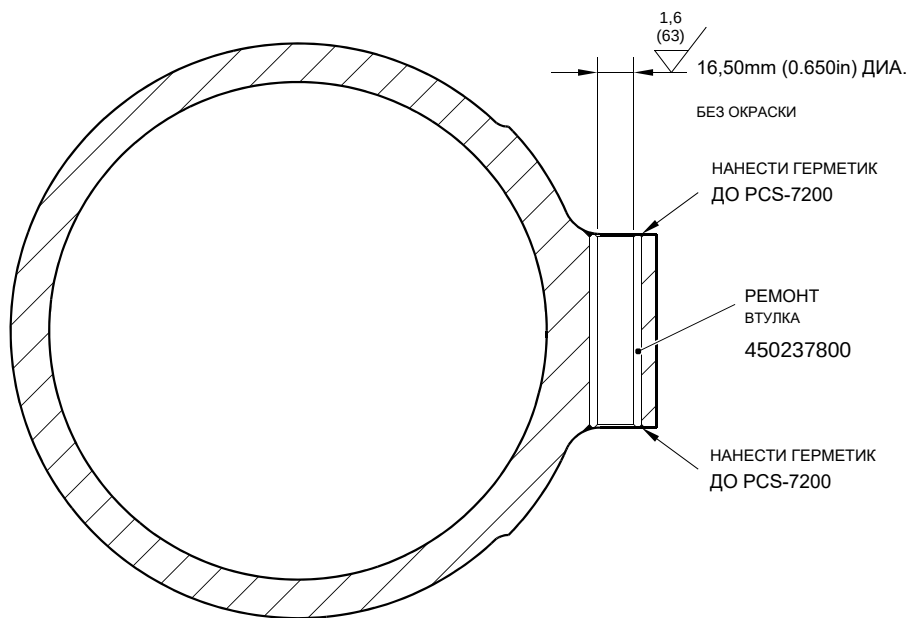
СЕЧЕНИЕ Z-Z
