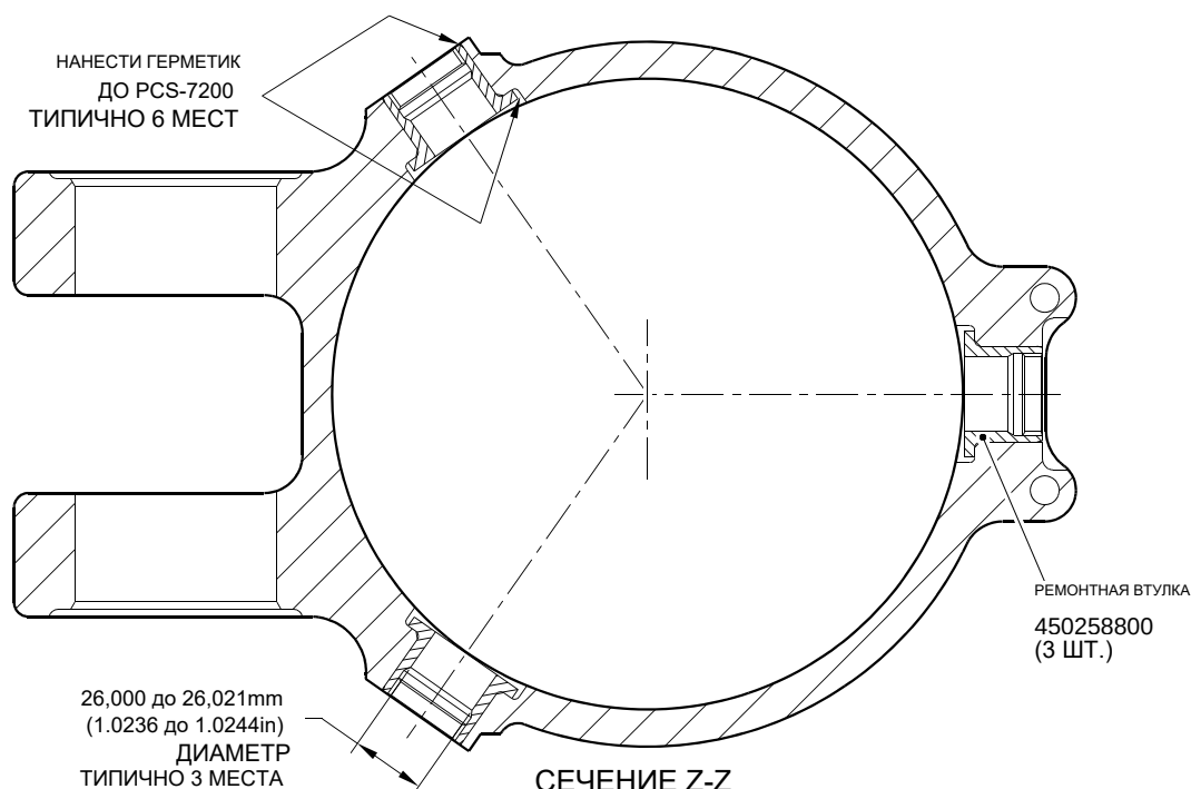
РЕМОНТНАЯ ВТУЛКА 450258800
