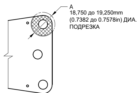
ВИД С
