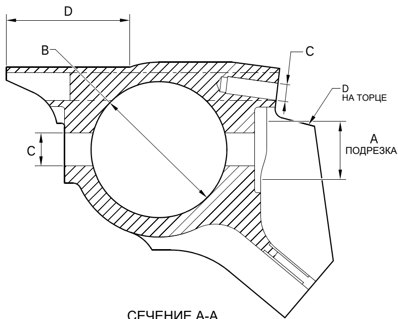
СЕЧЕНИЕ А-А
