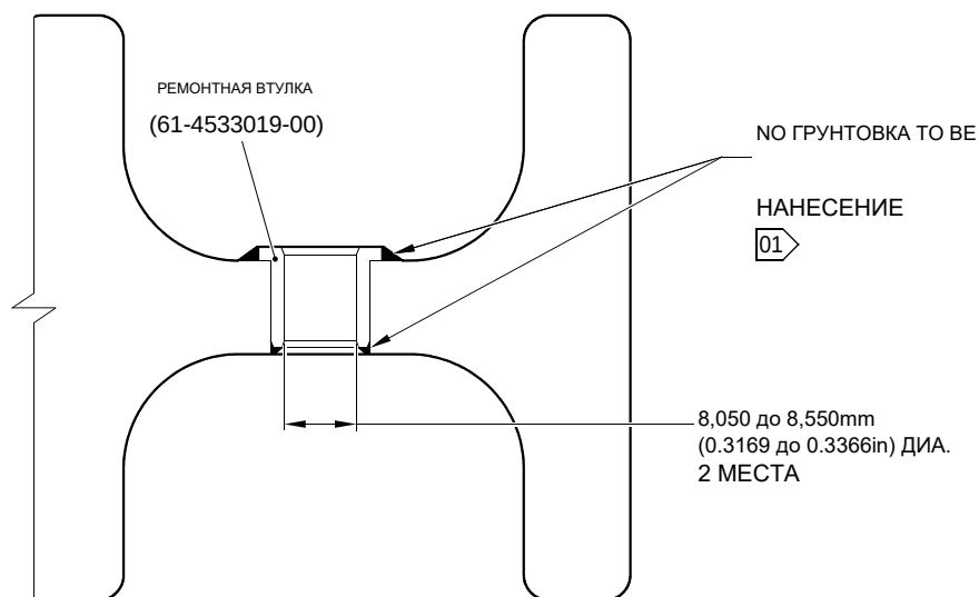
СЕЧЕНИЕ Y-Y (С ВЕРХНИМ)
