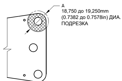
ВИД С
