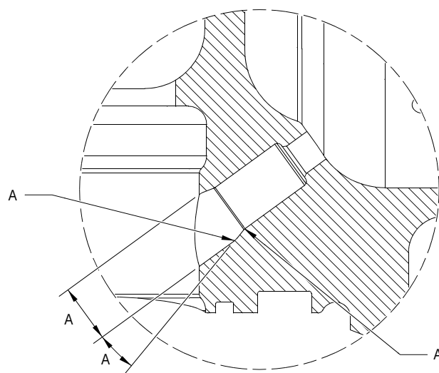
ДЕТАЛЬ Y
