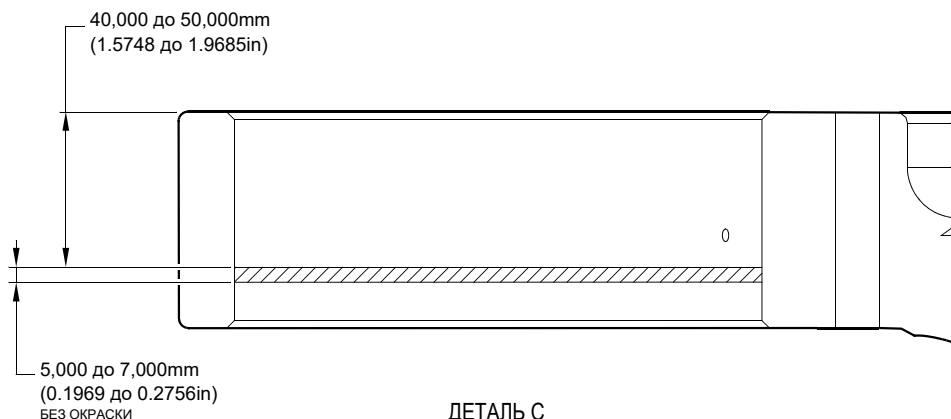
ДЕТАЛЬ С
