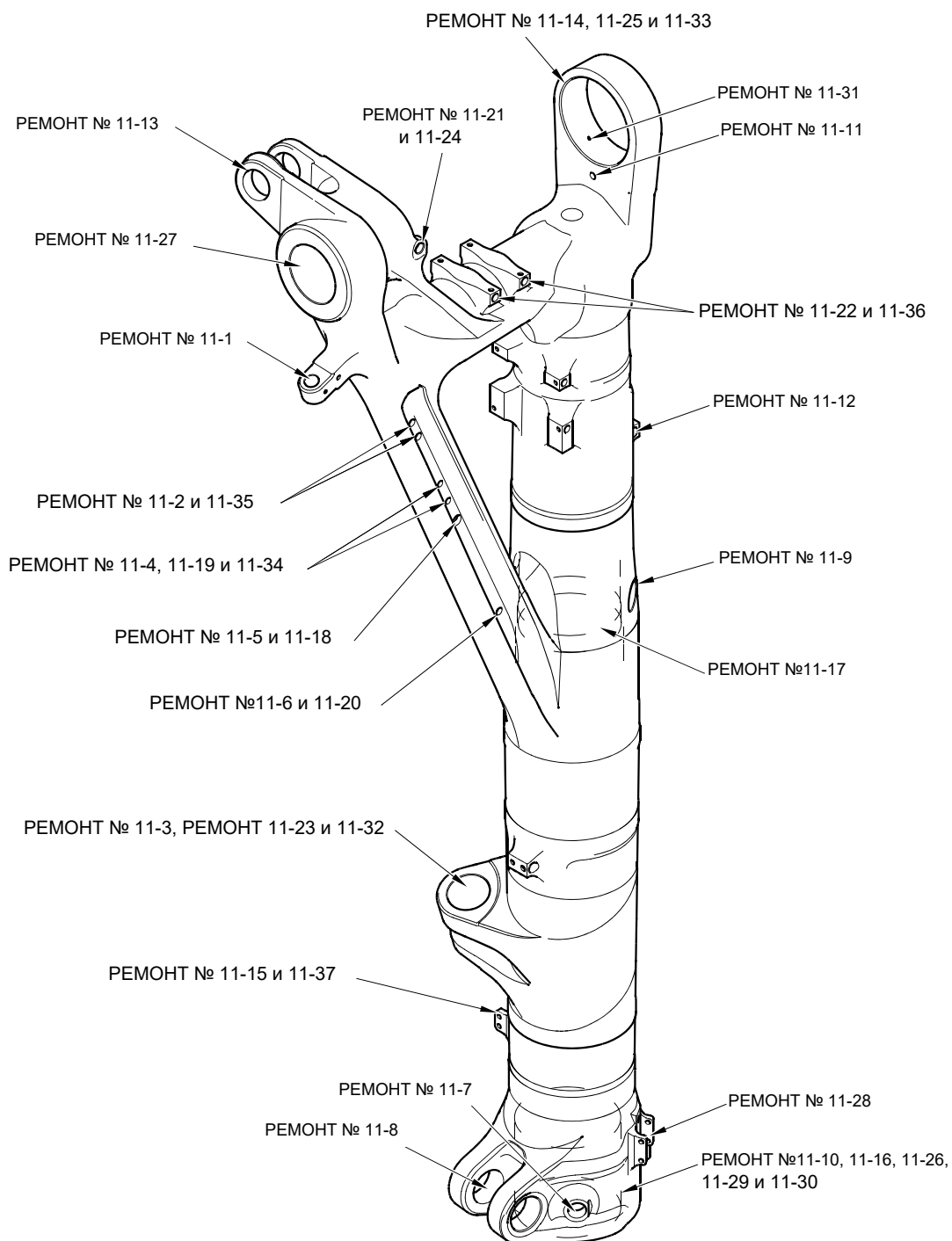
Ремонты корпуса стойки – Ключевая схема Рисунок 650
