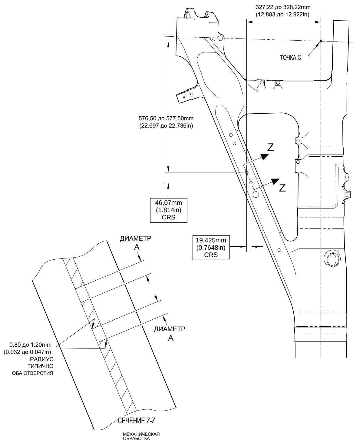
Ремонт корпуса стойки Рисунок 601
