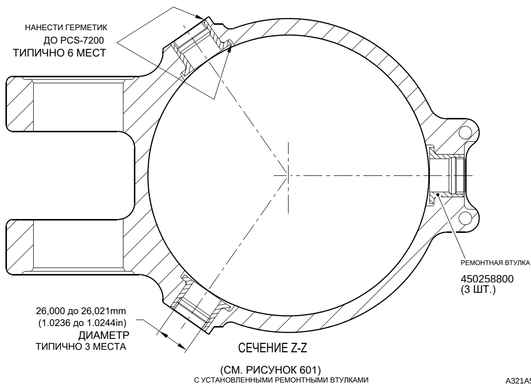
РЕМОНТНАЯ ВТУЛКА 450258800
