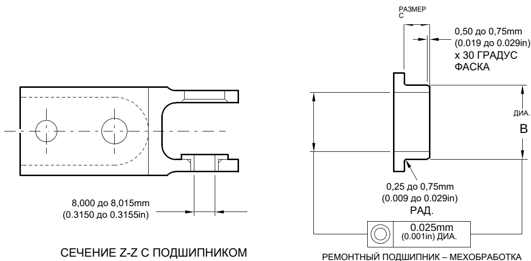
РЕМОНТНЫЙ ПОДШИПНИК – МЕХОБРАБОТКА
