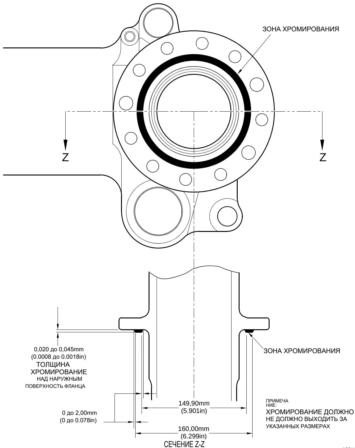
Ремонт скользящей трубы Рисунок 601
