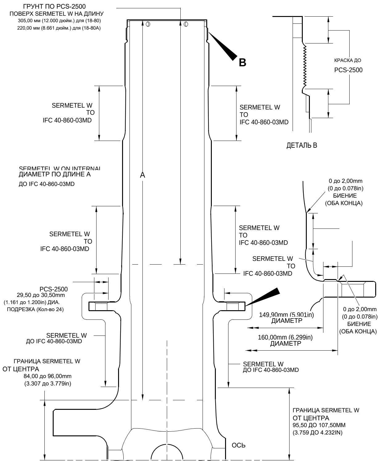
Скользкая труба (18-80) или (18-80A) – Защитная обработка Рисунок 618 – Лист 2
