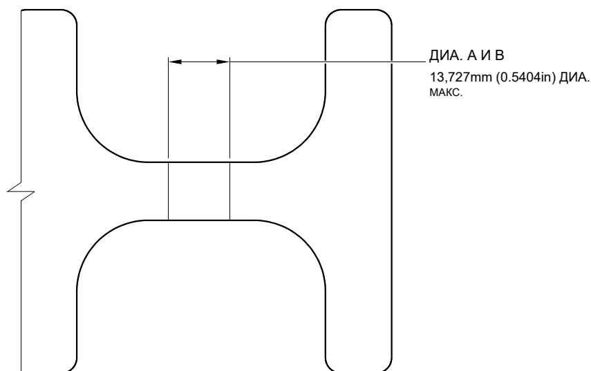
СЕЧЕНИЕ Y-Y (С ВТУЛКАМИ)
