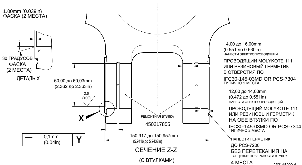
Ремонтные втулки – мехобработка и установка Рисунок 602
