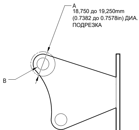
ВИД А
