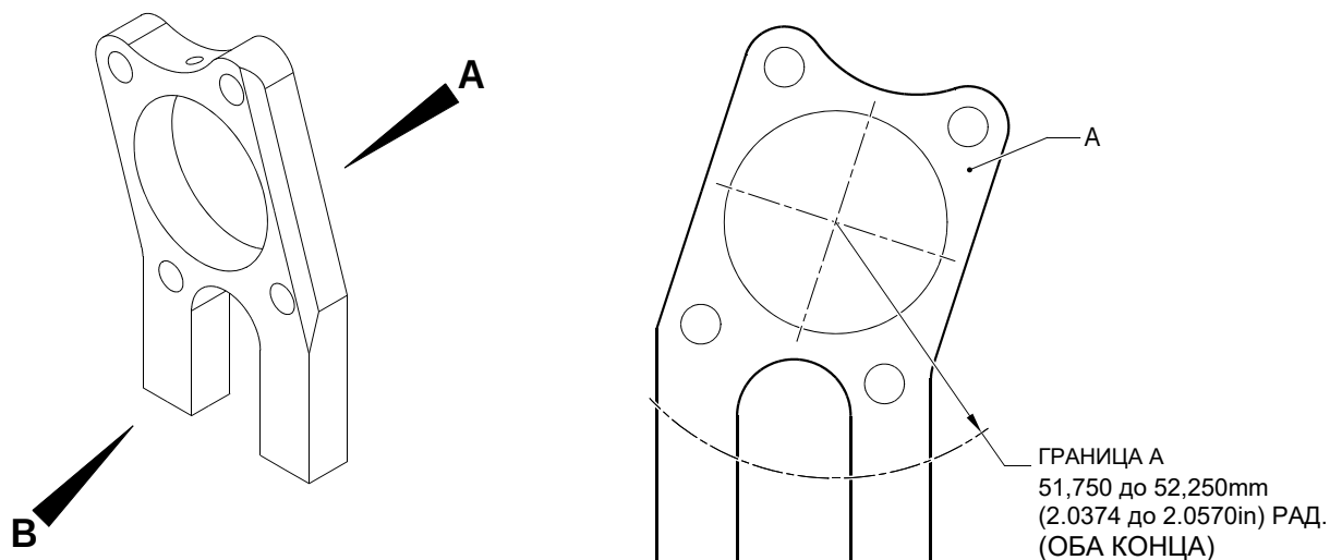
ВИД А
