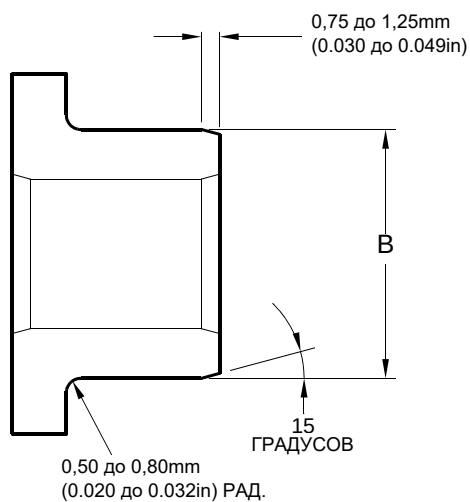
РЕМОНТНАЯ ВТУЛКА 450237819
