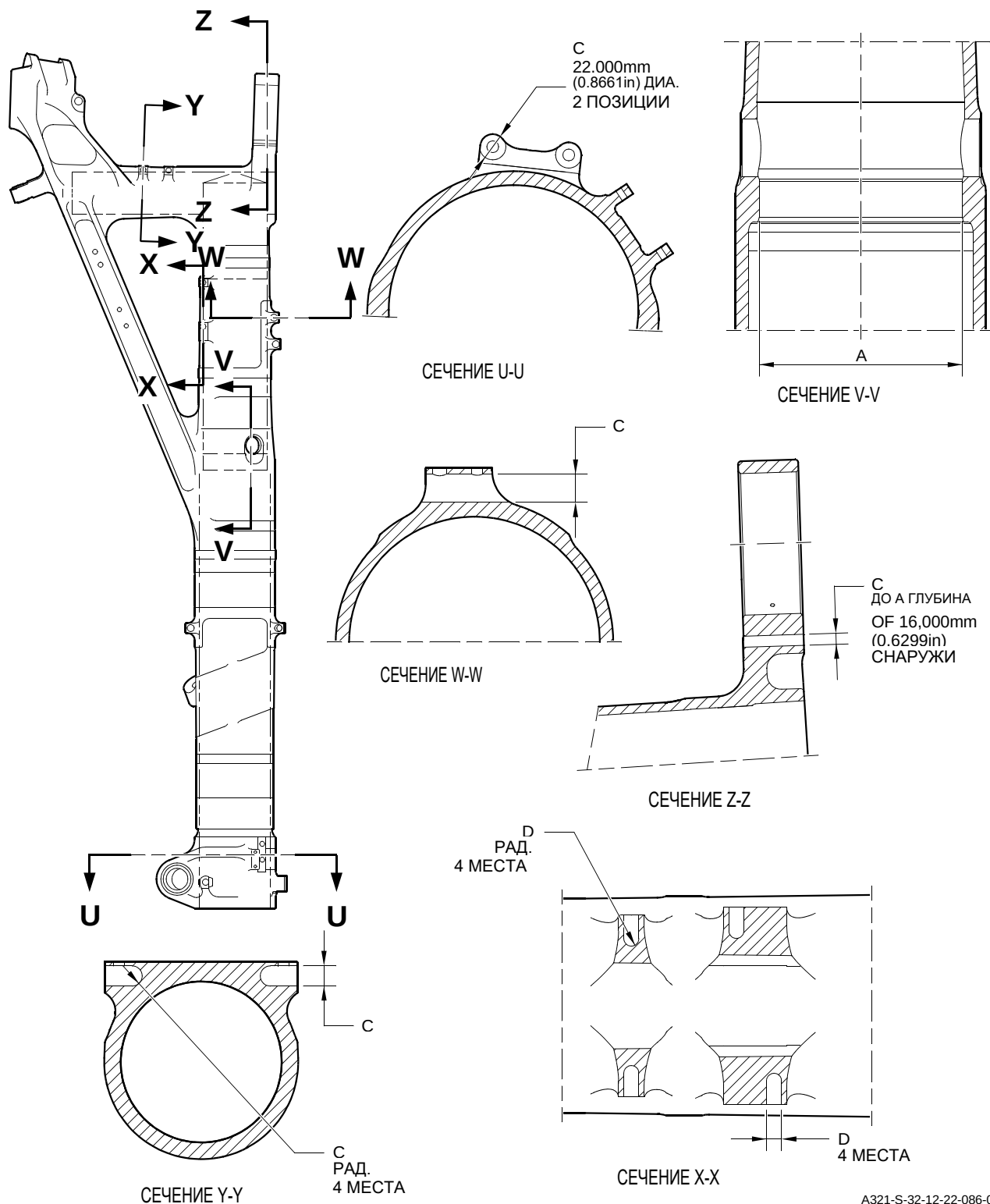
Корпус стойки (20-410А) и (20-420А) – Защитная обработка Рисунок 622 – Лист 2
