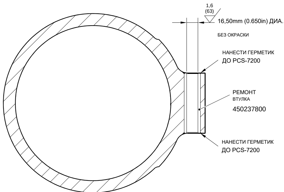
СЕЧЕНИЕ Z-Z
