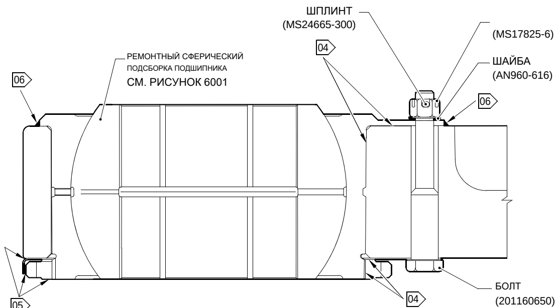
СЕЧЕНИЕ Z-Z
