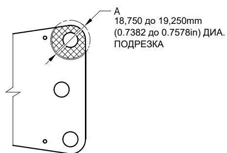
ВИД С
