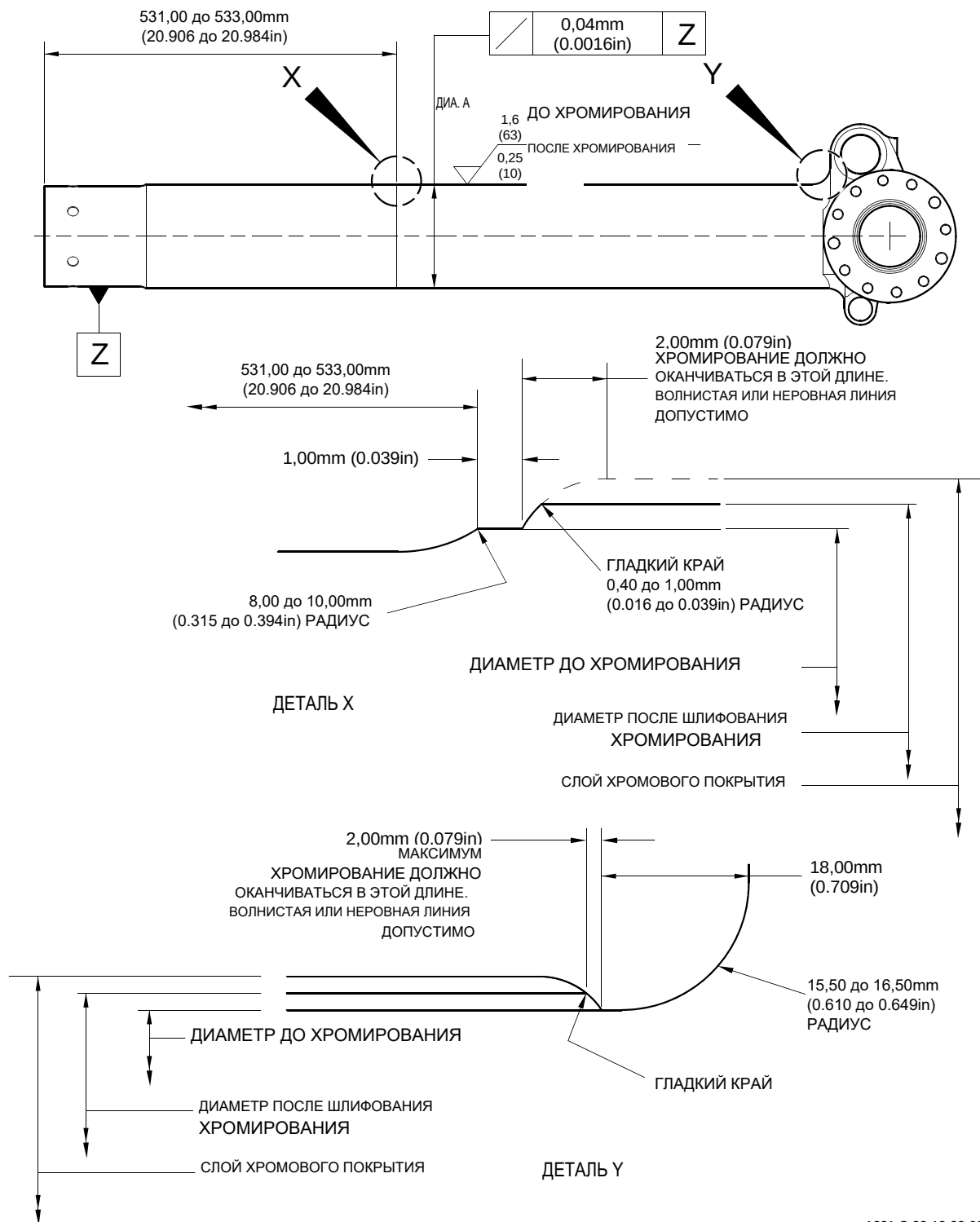
Ремонт скользящей трубы Рисунок 601
