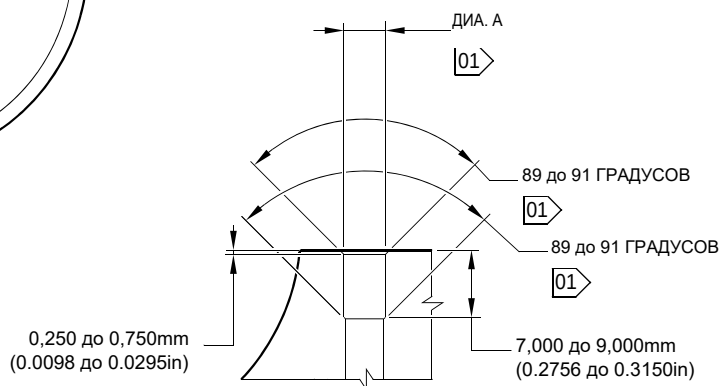
ДЕТАЛЬ С
