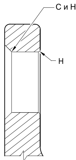
СЕЧЕНИЕ T-T ТИПОВО 12 МЕСТ
