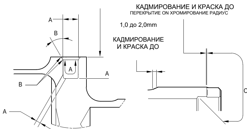
ДЕТАЛЬ W
