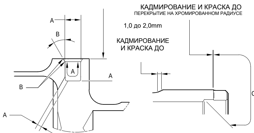
ДЕТАЛЬ W
