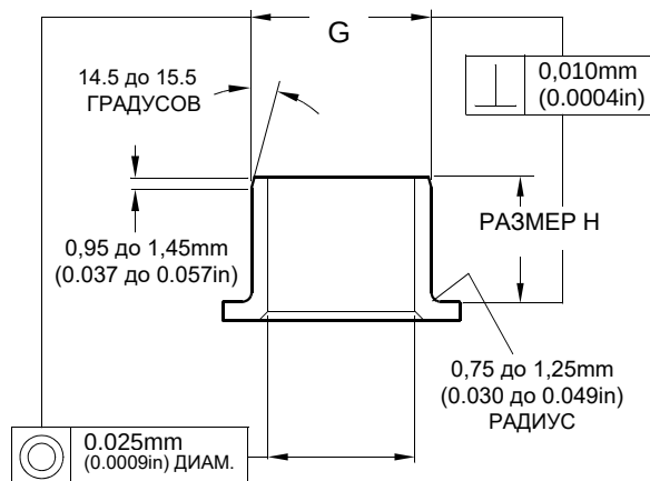
РЕМОНТНЫЙ ПОДШИПНИК 450258810
