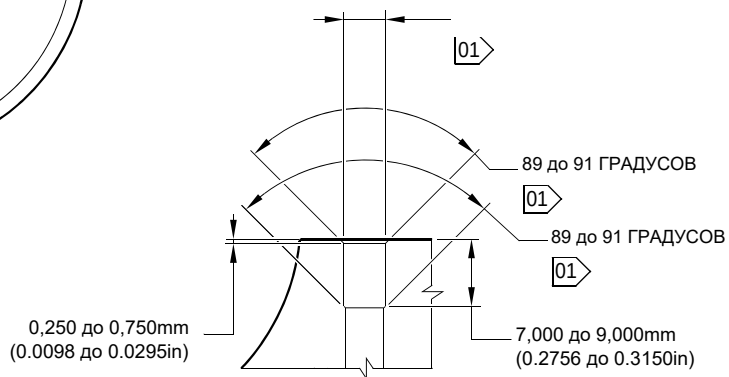
СЕЧЕНИЕ Y-Y (БЕЗ СМАЗОЧНОГО АДАПТЕРА)
