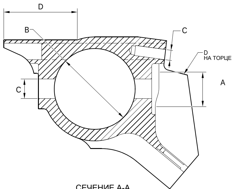
СЕЧЕНИЕ А-А
