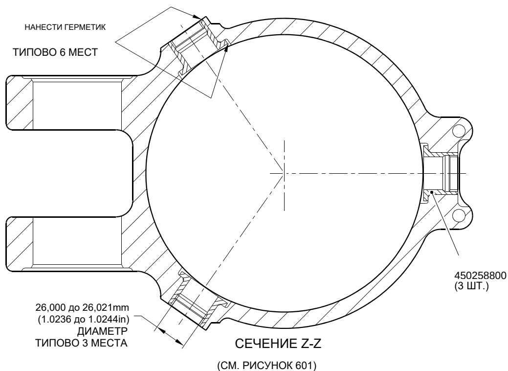
РЕМОНТНАЯ ВТУЛКА 450258800
