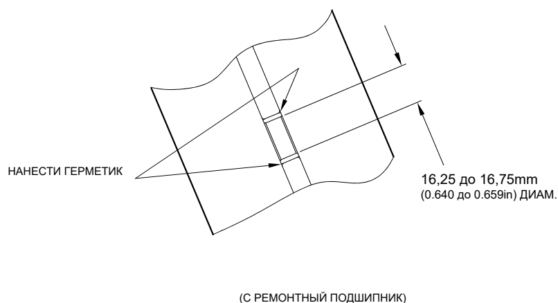
(С РЕМОНТНЫЙ ПОДШИПНИК)
