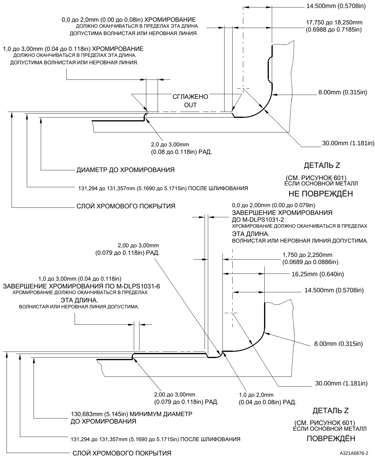
Ремонт скользящей трубы Рисунок 602
