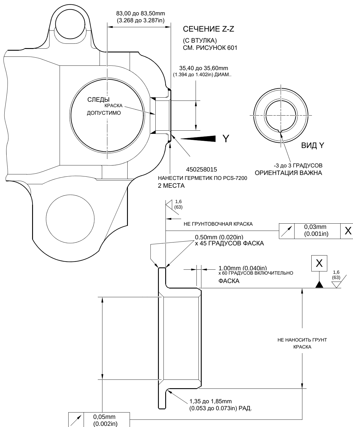
РЕМОНТНАЯ ВТУЛКА 450258015
