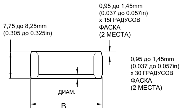
РЕМОНТНЫЙ ПОДШИПНИК
