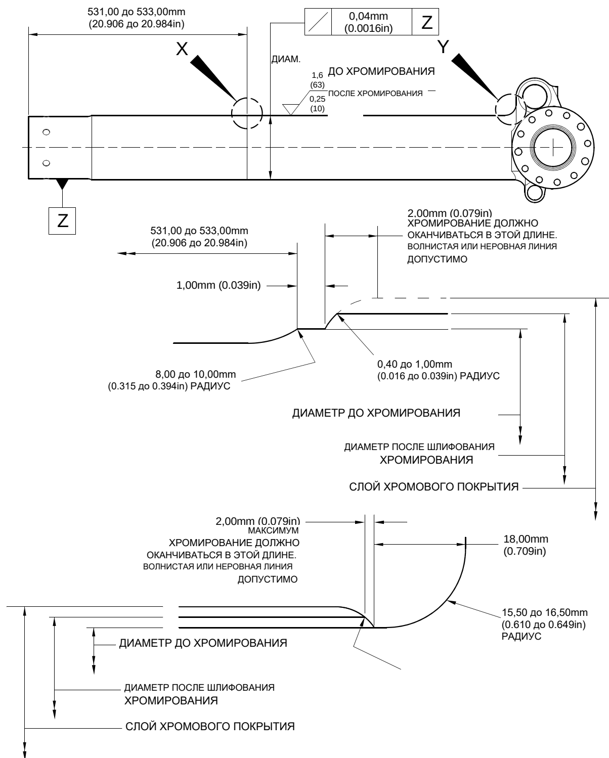
Ремонт скользящей трубы Рисунок 601
