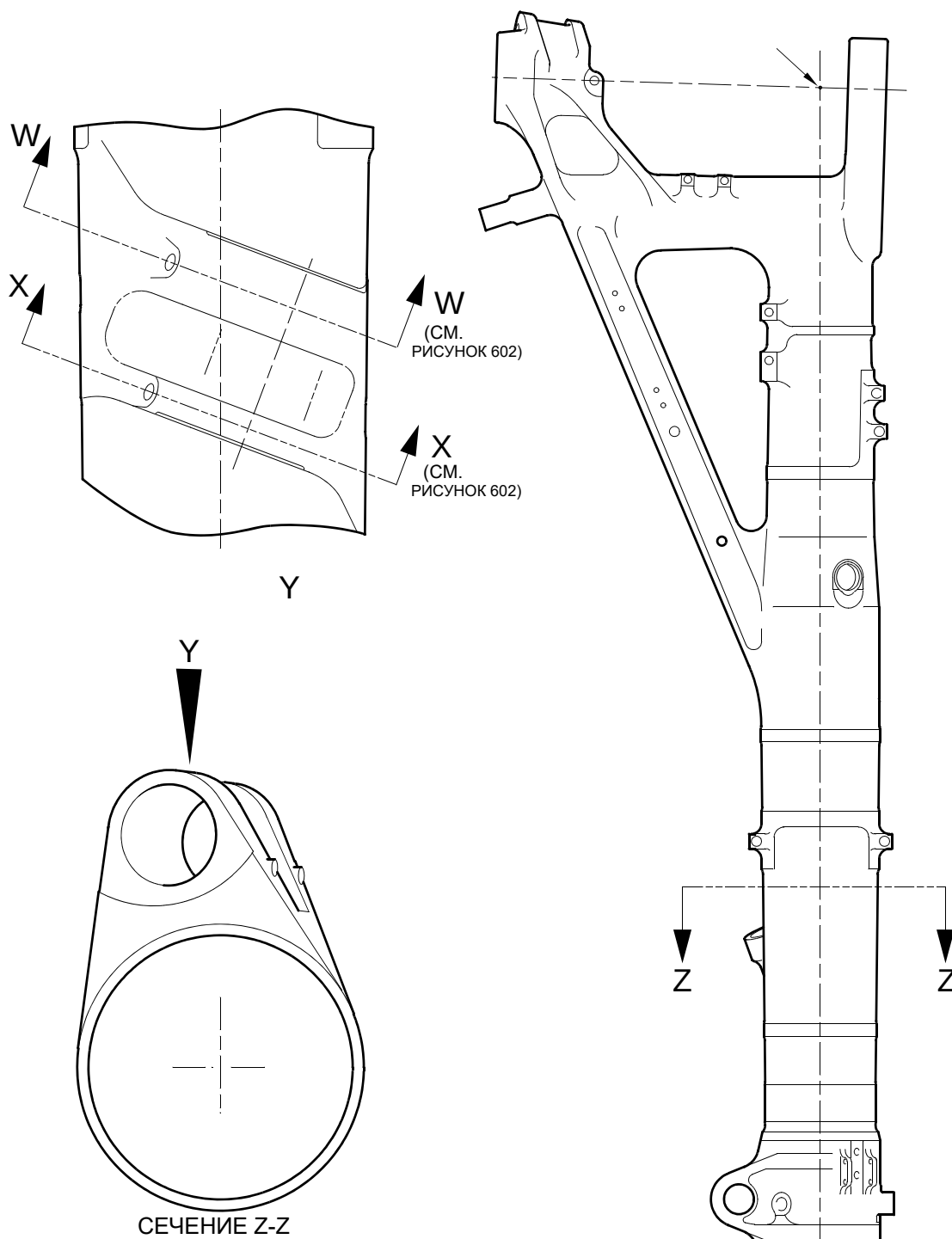
Ремонт корпуса стойки Рисунок 601
