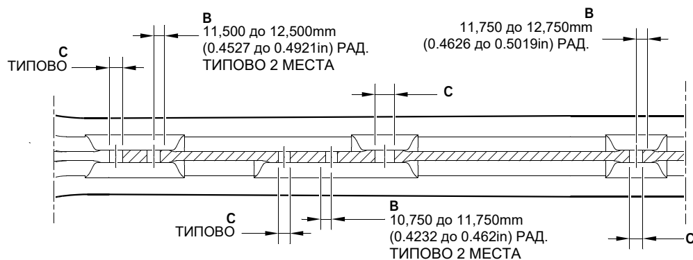
СЕЧЕНИЕ В-В ОТВЕРСТИЯ ПОДКОСА ТОЛЬКО ДЛЯ КОРПУСА СТОЙКИ (20-410C, 20-420C)
