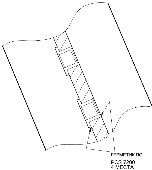
С РЕМОНТНЫМИ ВТУЛКАМИ
