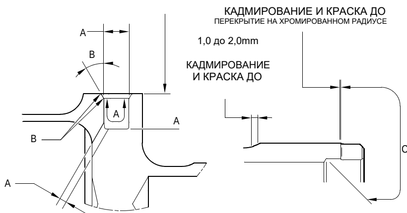
ДЕТАЛЬ W
