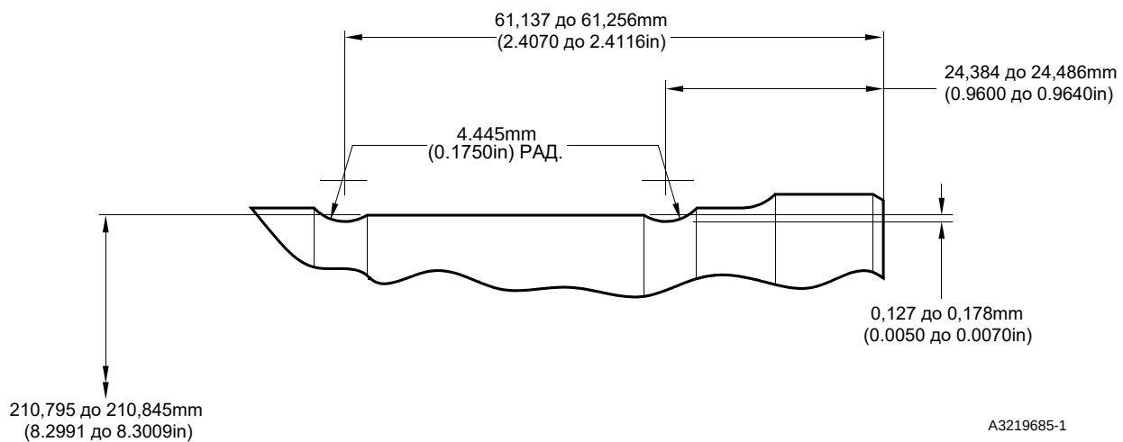
Ремонт подсорки нижнего подшипника Рисунок 601
