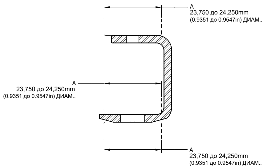
СЕЧЕНИЕ Z-Z
