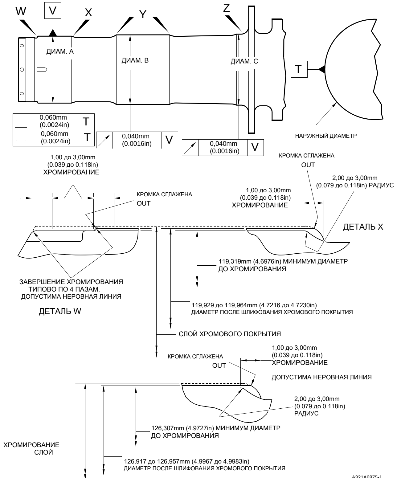
Ремонт скользящей трубы Рисунок 601
