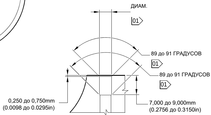
СЕЧЕНИЕ Y-Y (БЕЗ СМАЗОЧНОГО АДАПТЕРА)
