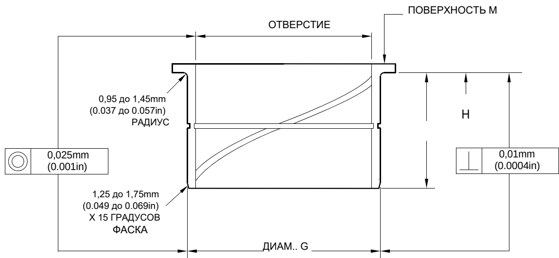
РЕМОНТНАЯ ВТУЛКА 450258806 МЕХАНИЧЕСКАЯ ОБРАБОТКА
