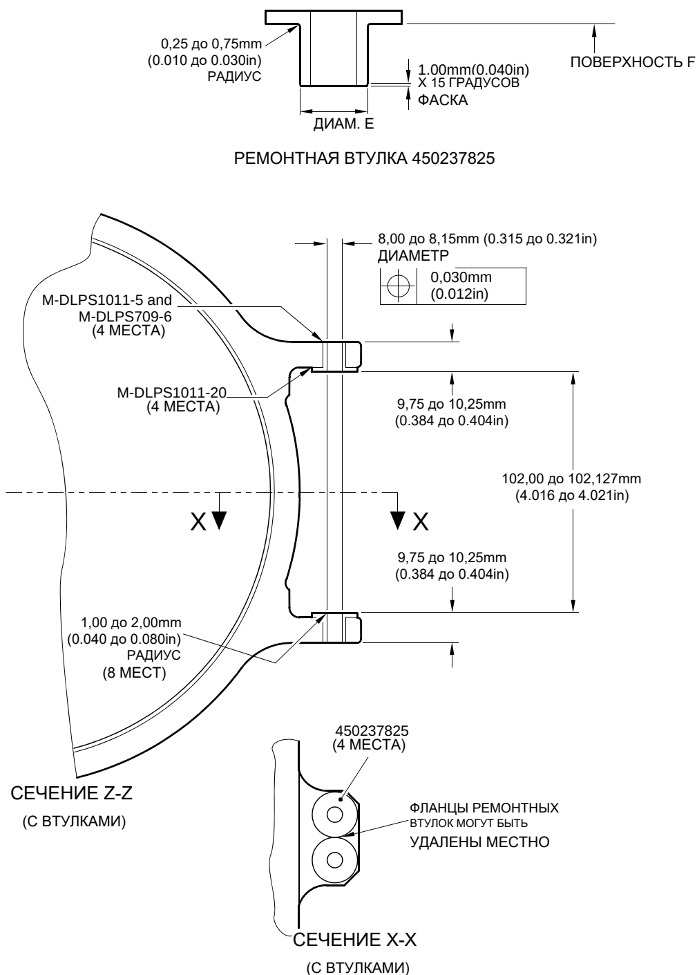
Ремонтная втулка – мехобработка и установка Рисунок 603
