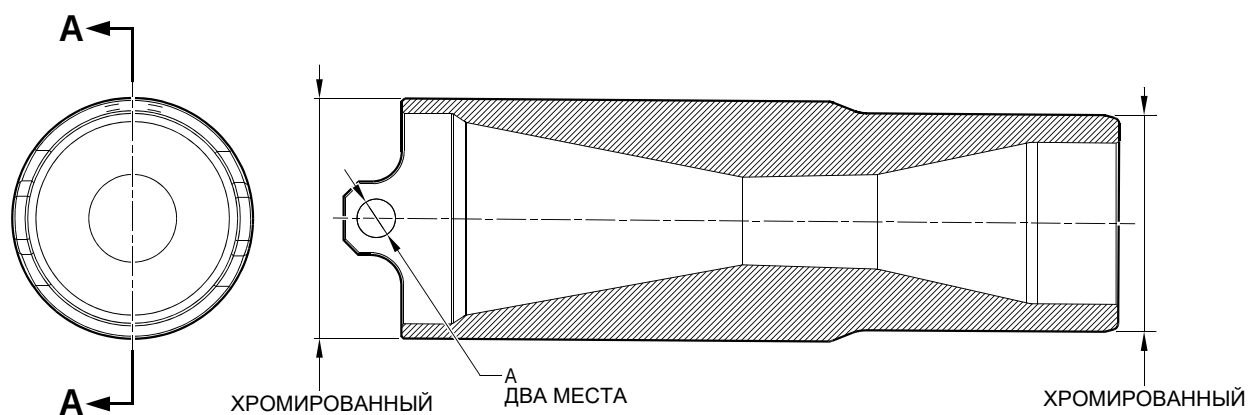
СЕЧЕНИЕ А-А
