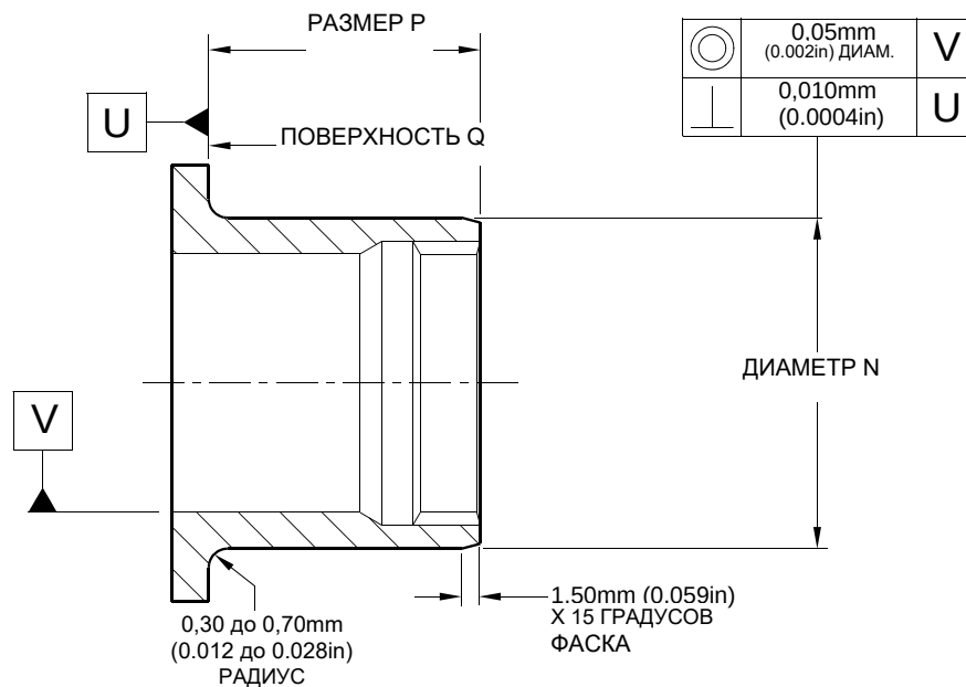
РЕМОНТНАЯ ВТУЛКА 450258800
