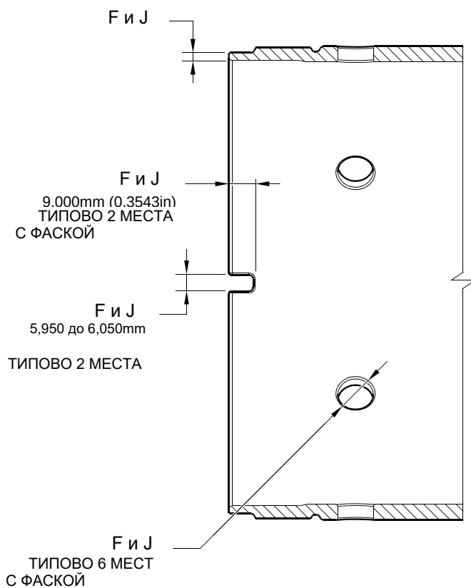
СЕЧЕНИЕ U-U СТВОЛ
