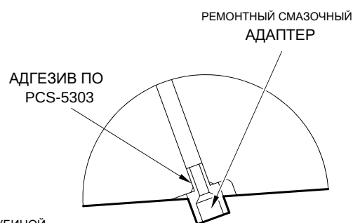
ДЕТАЛЬ Y (С СМАЗОЧНЫМ АДАПТЕРОМ)
