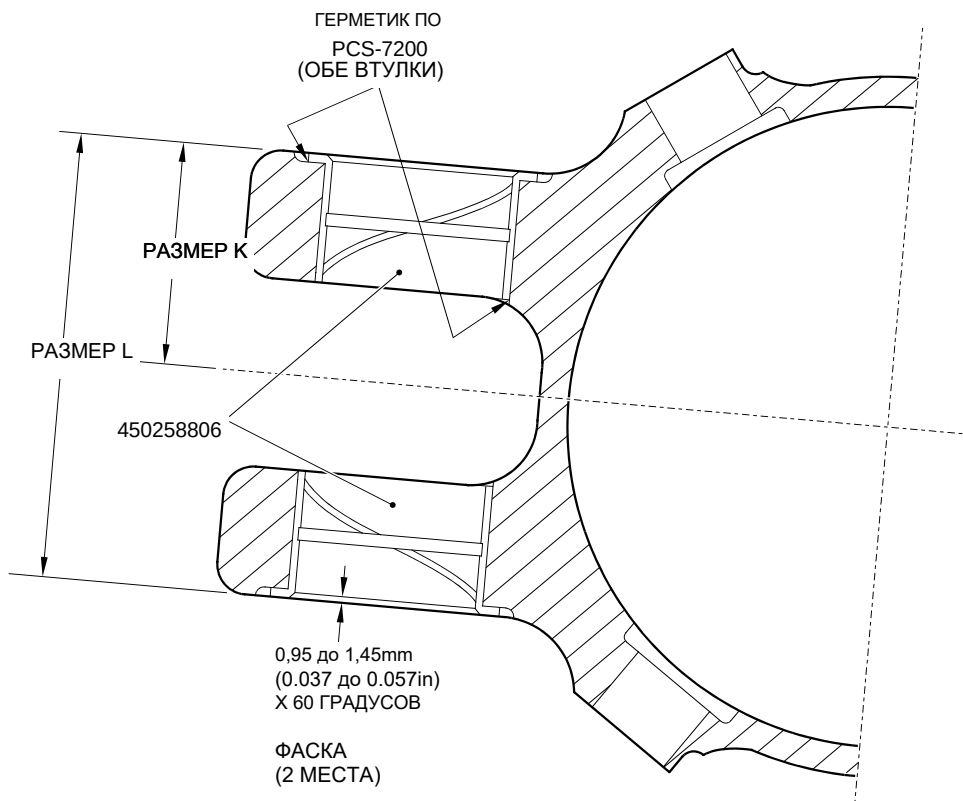
РЕМОНТНАЯ ВТУЛКА 450258806 МЕХАНИЧЕСКАЯ ОБРАБОТКА
