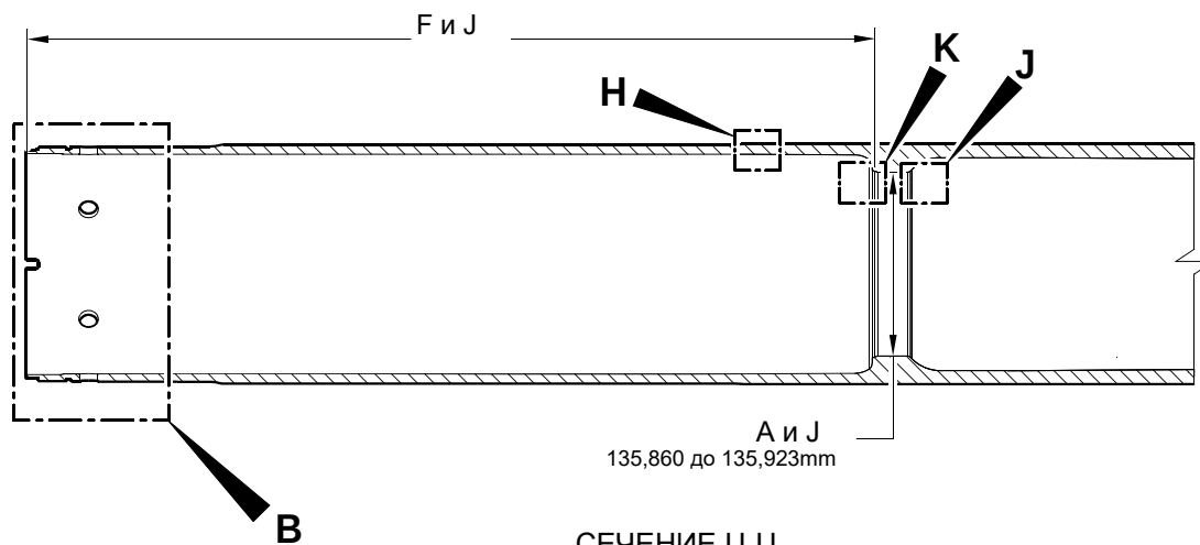
СЕЧЕНИЕ U-U СТВОЛ
