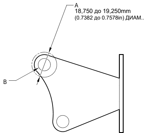
ВИД А
