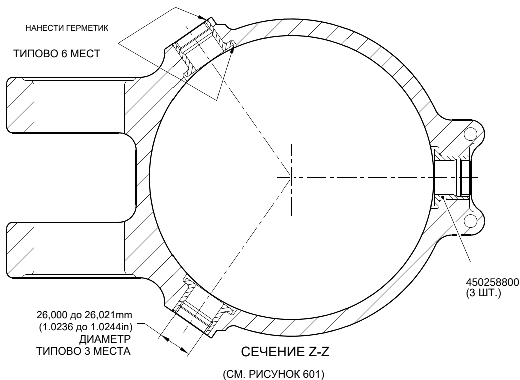
РЕМОНТНАЯ ВТУЛКА 450258800
