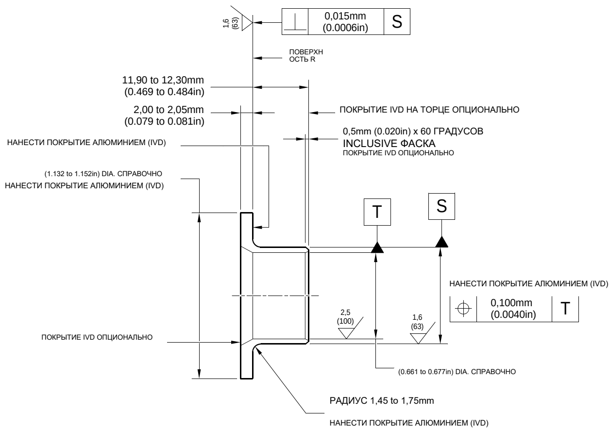
РАЗРЕЗ W-W (С ВТУЛКАМИ)
