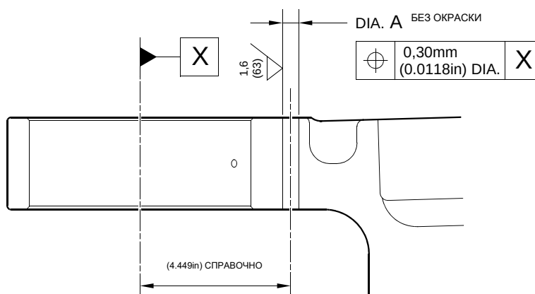
РАЗРЕЗ Z-Z (БЕЗ ПОДШИПНИКА)
