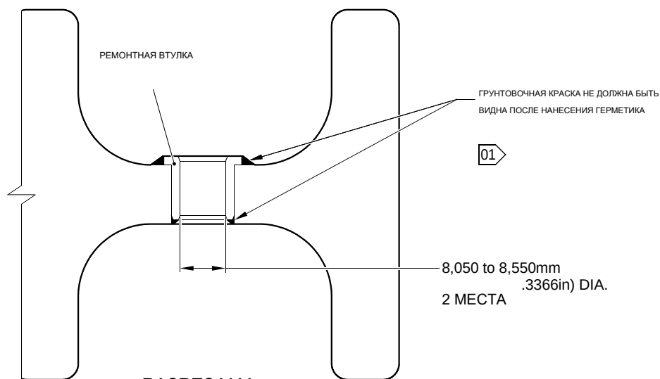
РАЗРЕЗ Y-Y (С ВТУЛКАМИ)
