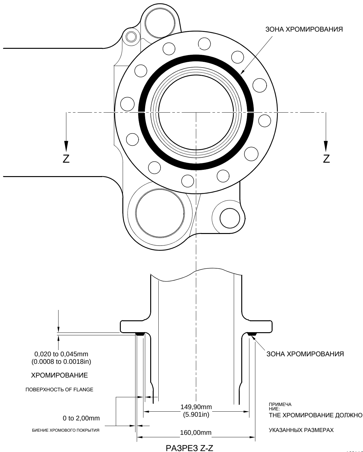
Ремонт скользящей трубы Рисунок 601
