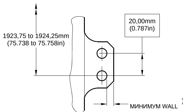
РАЗРЕЗ X-X (БЕЗ ВТУЛОК)
