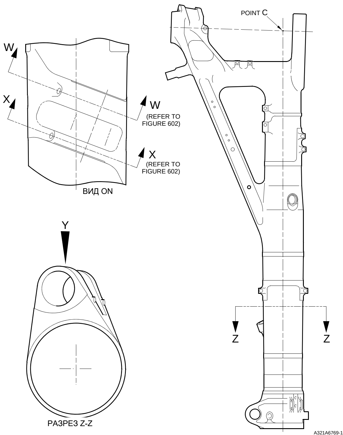
Ремонт корпуса стойки Рисунок 601
