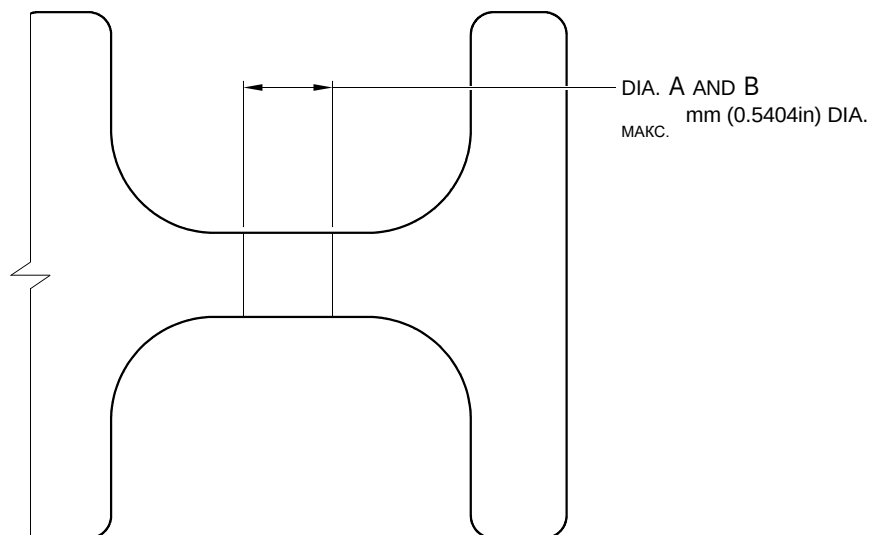
РАЗРЕЗ Y-Y (БЕЗ ВТУЛОК)
