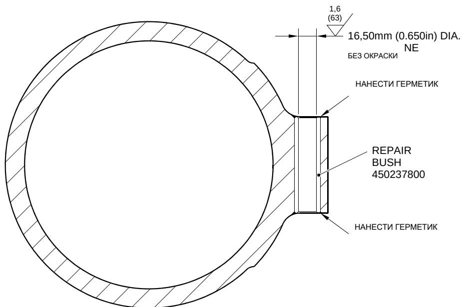
РАЗРЕЗ Z-Z
