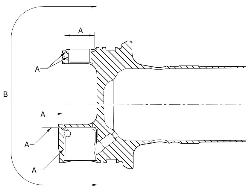
РАЗРЕЗ A-A
