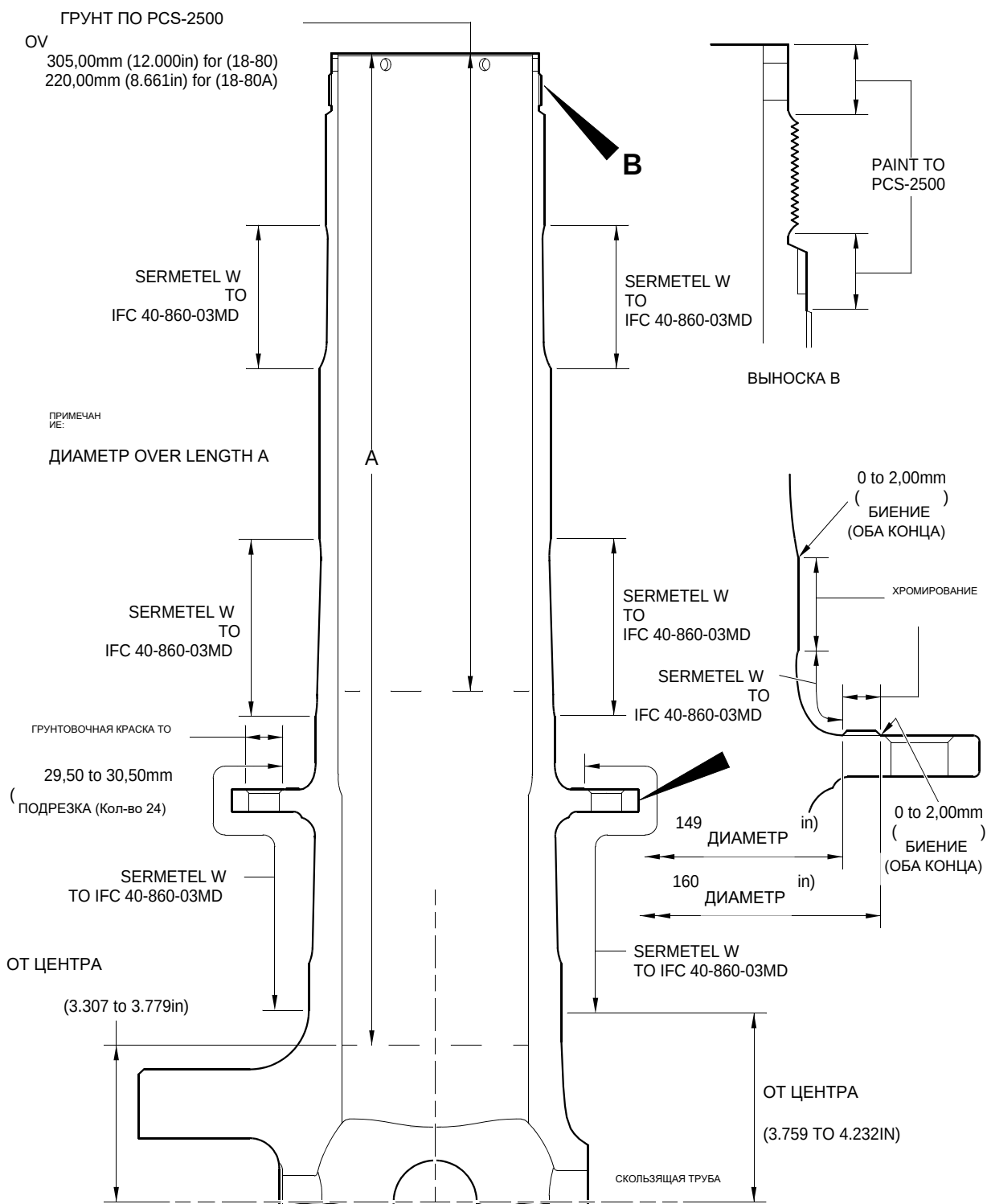
Скользкая труба (18-80) или (18-80А) – Защитная обработка Рисунок 618 – Лист 2
