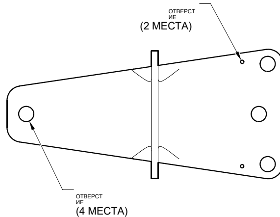
ВИД А
