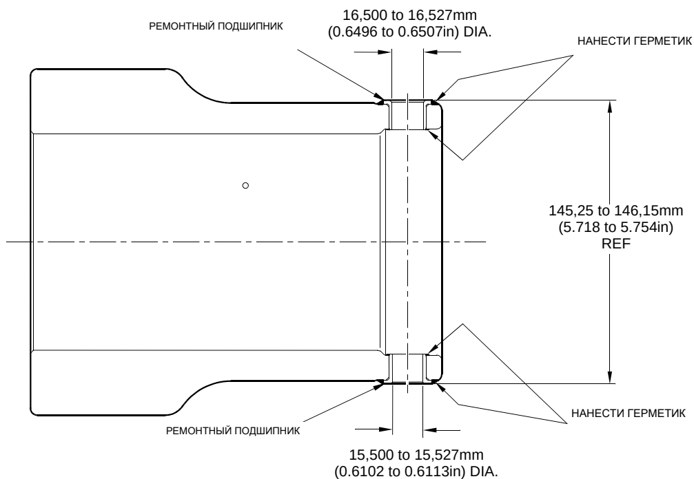
РАЗРЕЗ Z-Z (СМ. РИСУНОК 601)
