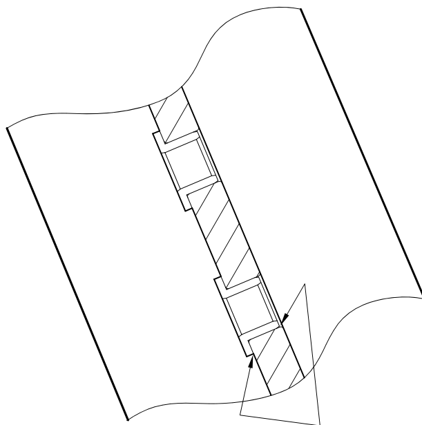
PART РАЗРЕЗ Z-Z С РЕМОНТНЫМИ ВТУЛКАМИ
