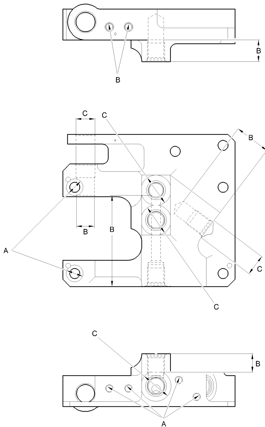
Переходной блок (2-340, 2-340A, 2-350 и 2-350A) – Защитная обработка Рисунок 602
