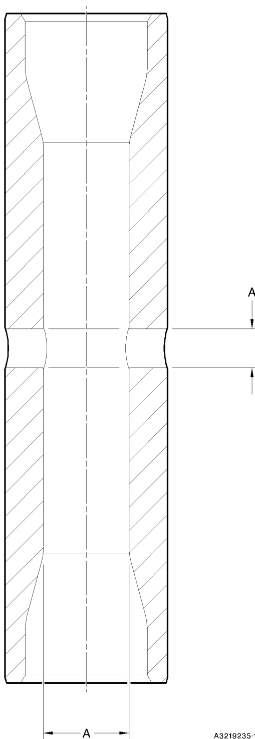
Штифт (11-130) – Защитная обработка Рисунок 610
