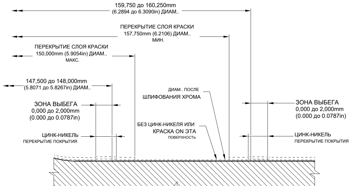
ДЕТАЛЬ Е
