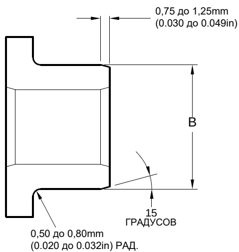
РЕМОНТНАЯ ВТУЛКА 450237819
