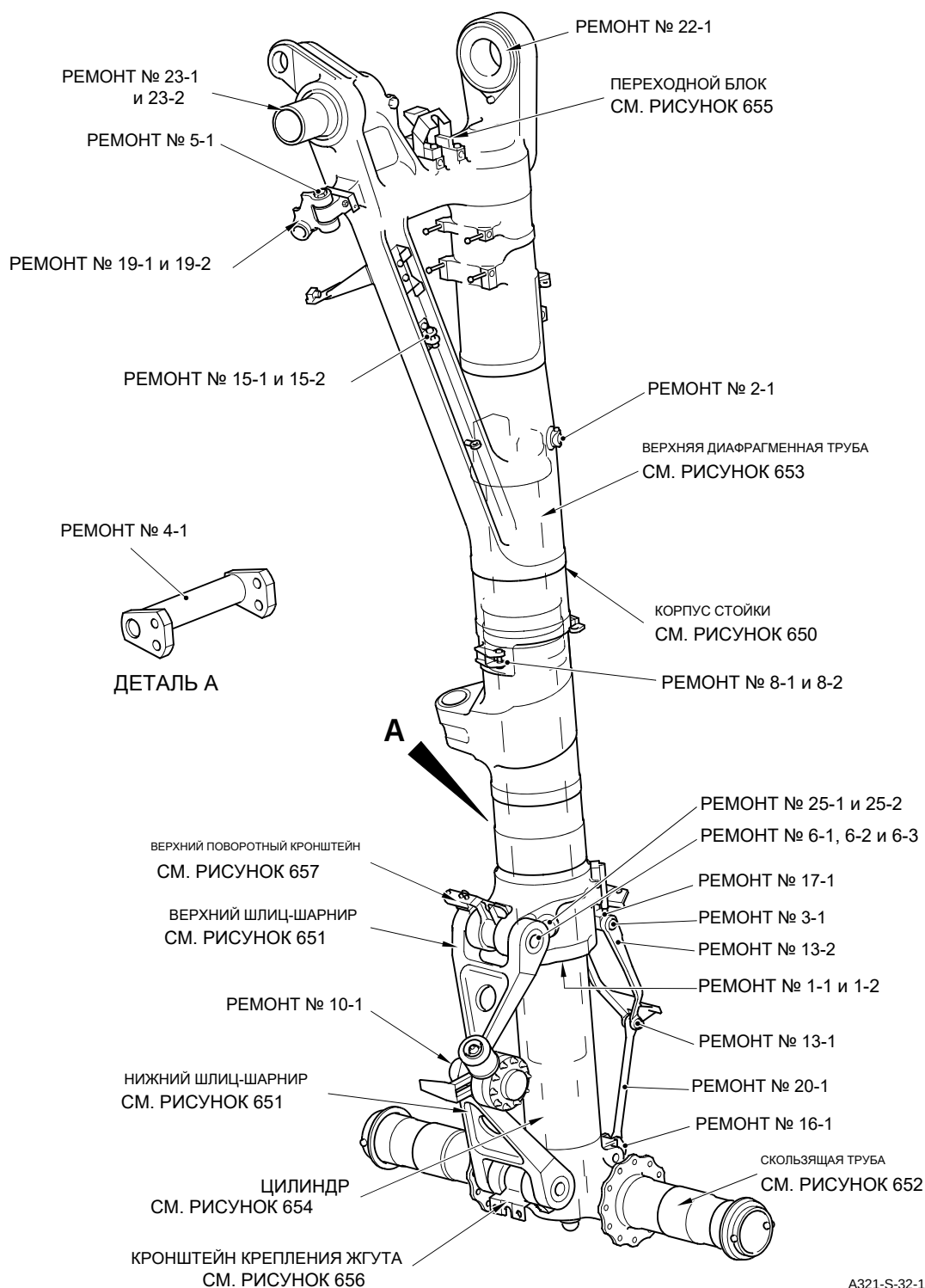
Допустимые ремонты – Ключевая схема Рисунок 649
