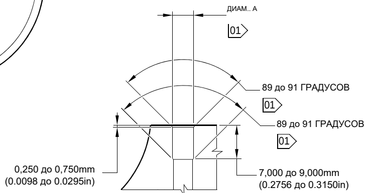
ДЕТАЛЬ С
