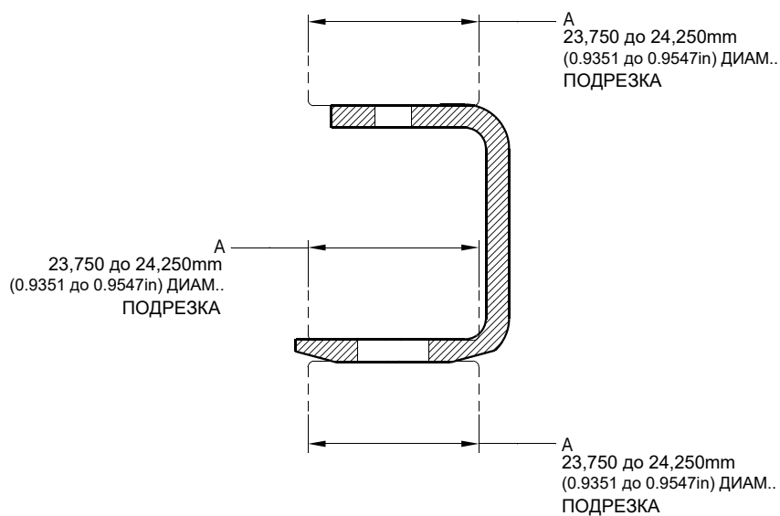
СЕЧЕНИЕ Z-Z
