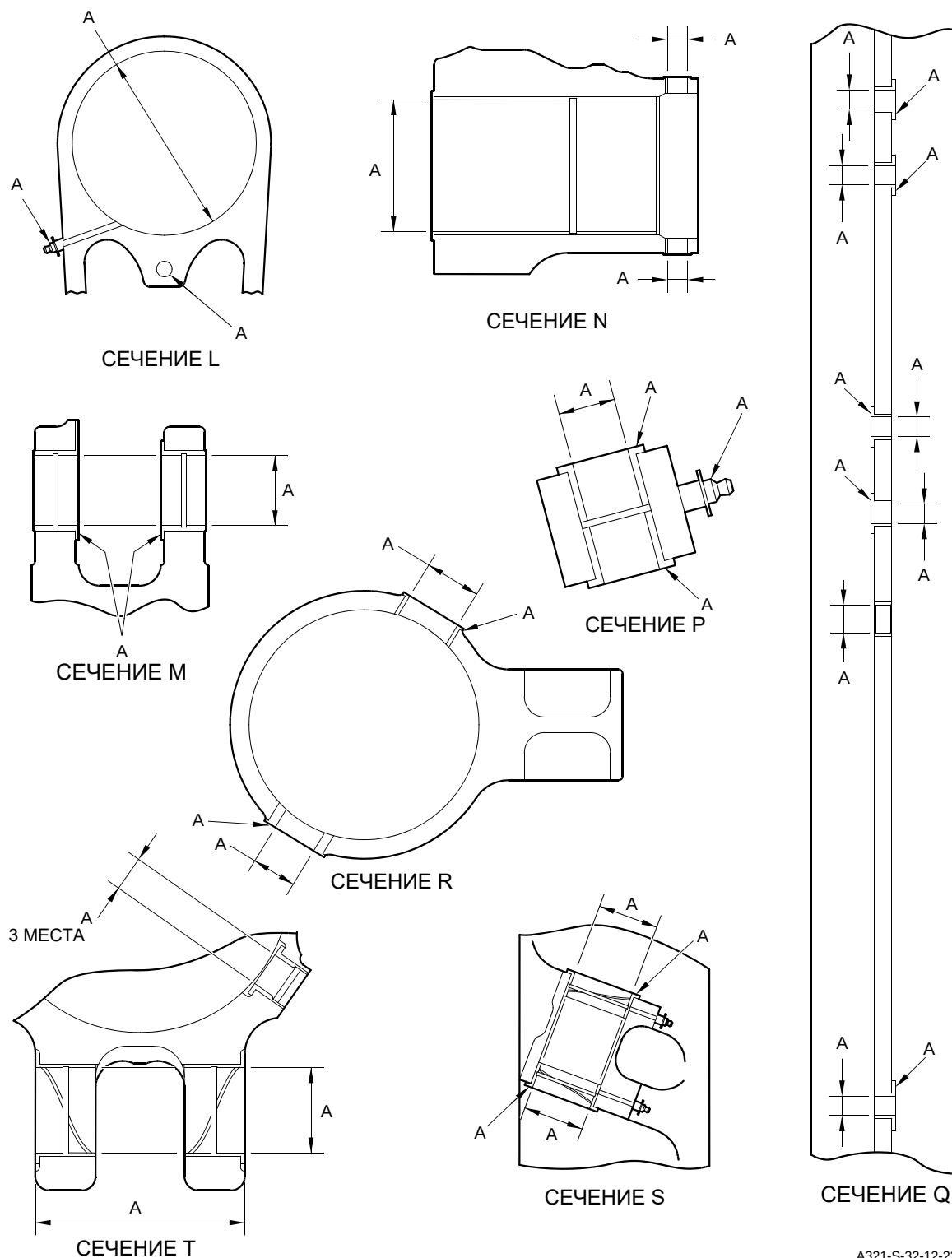
Подсборка корпуса стойки (20-90, 20-90A, 20-100 и 20-100A) – Защитная обработка Рисунок 619 – Лист 2
