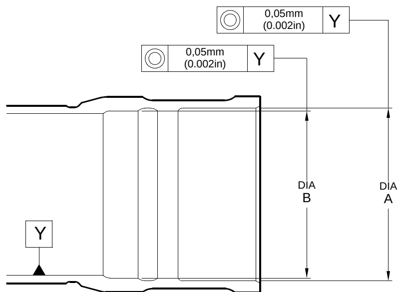
СЕЧЕНИЕ Z-Z
