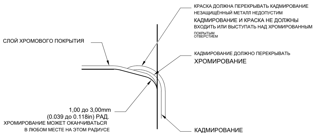
ДЕТАЛЬ W
