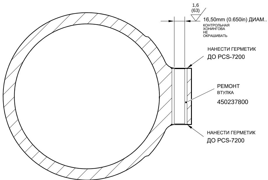
СЕЧЕНИЕ Z-Z
