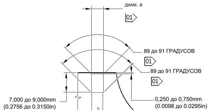
ДЕТАЛЬ В
