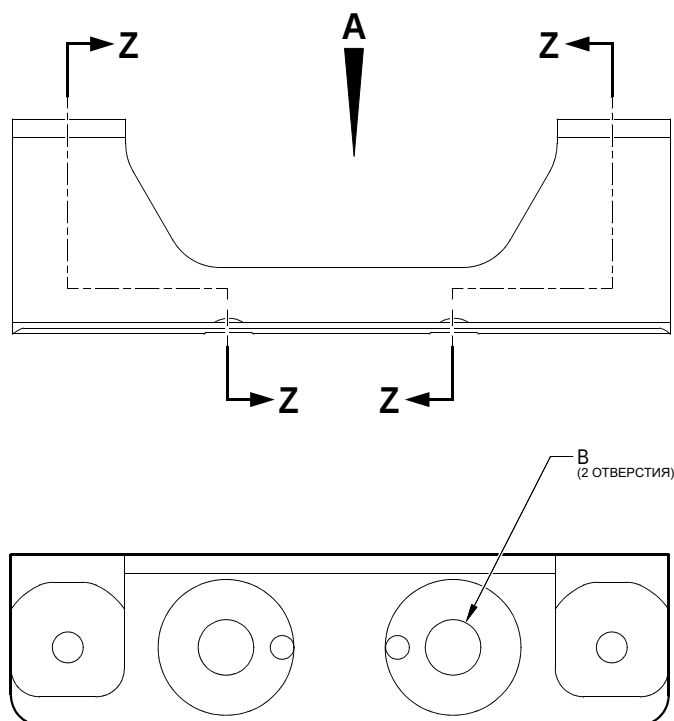
ВИД А
