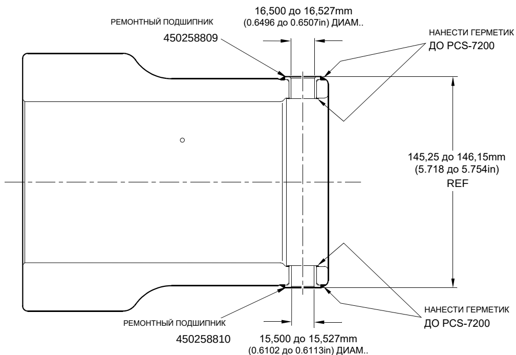
СЕЧЕНИЕ Z-Z (СМ. РИСУНОК 601)
