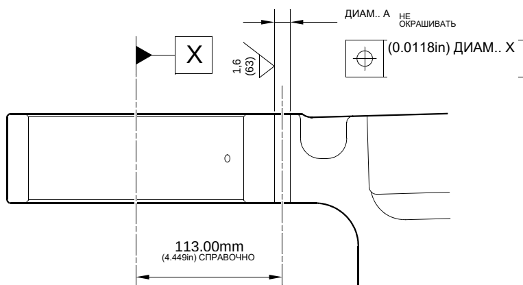
СЕЧЕНИЕ Z-Z (БЕЗ ПОДШИПНИКА)
