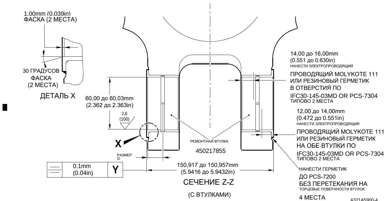
Ремонтные втулки – мехобработка и установка Рисунок 602
