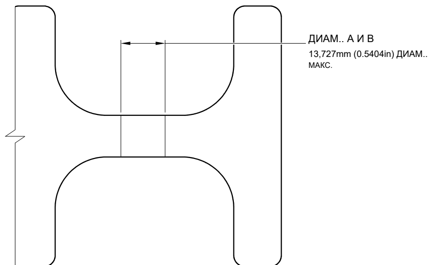
СЕЧЕНИЕ Y-Y (С ВЕРХНИМ)
