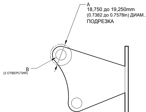
ВИД А
