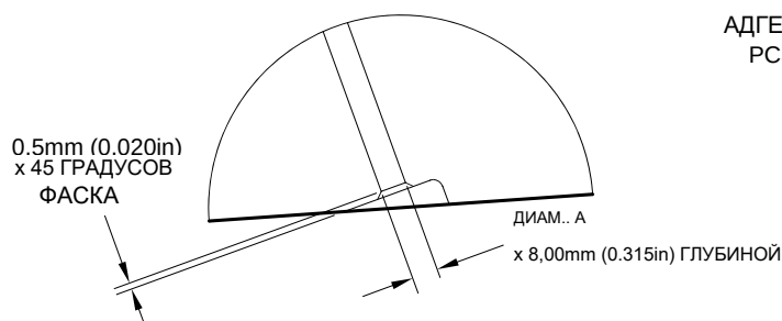
ДЕТАЛЬ Y (БЕЗ СМАЗОЧНОГО АДАПТЕРА)
