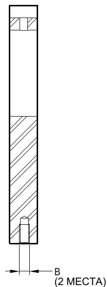
СЕЧЕНИЕ Z-Z
