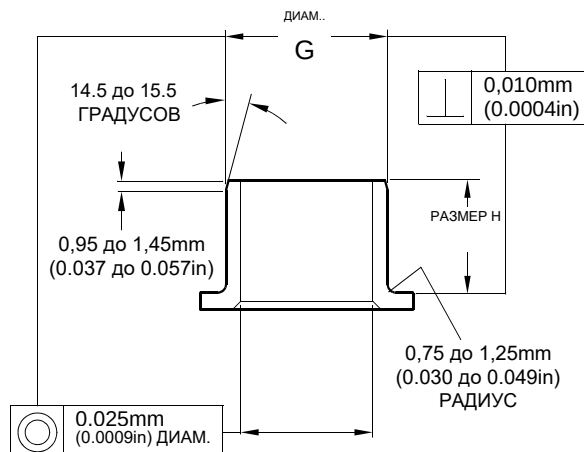
РЕМОНТНЫЙ ПОДШИПНИК 450258810
