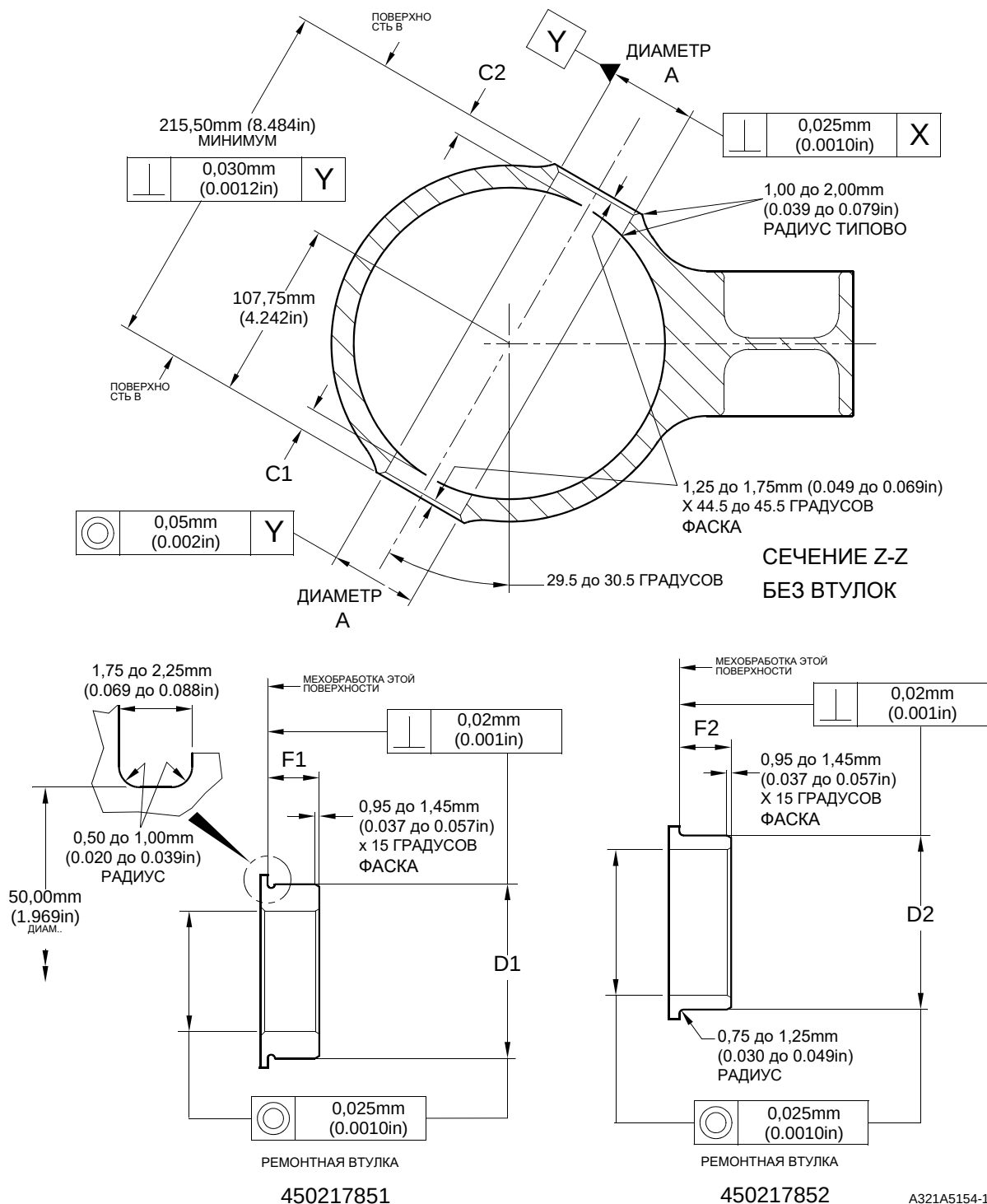
Ремонт корпуса стойки – мехобработка Рисунок 602
