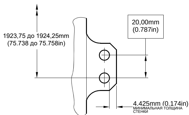
СЕЧЕНИЕ X-X (БЕЗ ВТУЛОК)
