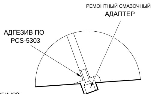
ДЕТАЛЬ Y (С СМАЗОЧНЫМ АДАПТЕРОМ)
