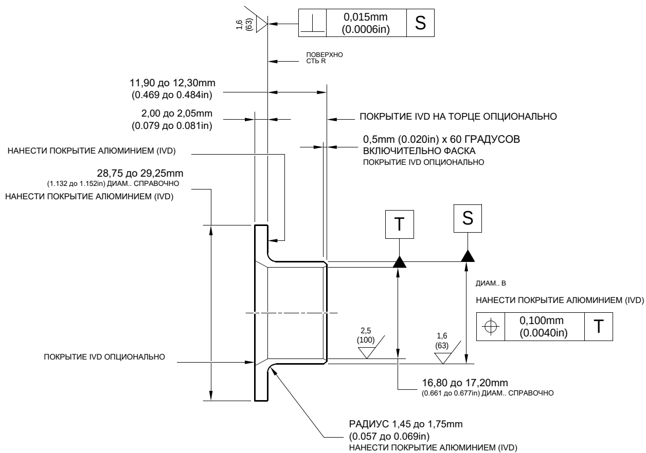
СЕЧЕНИЕ W-W (С ВТУЛКАМИ)
