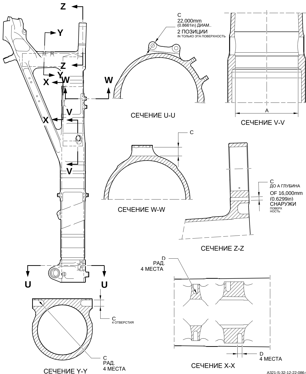
Корпус стойки (20-410A) и (20-420A) – Защитная обработка Рисунок 622 – Лист 2
