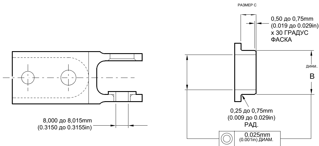
РЕМОНТНЫЙ ПОДШИПНИК – МЕХОБРАБОТКА
