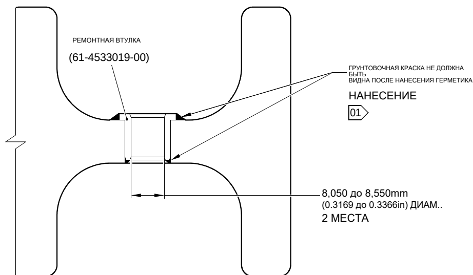
СЕЧЕНИЕ Y-Y (С ВЕРХНИМ)
