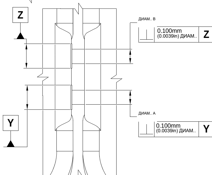
СЕЧЕНИЕ Z-Z
