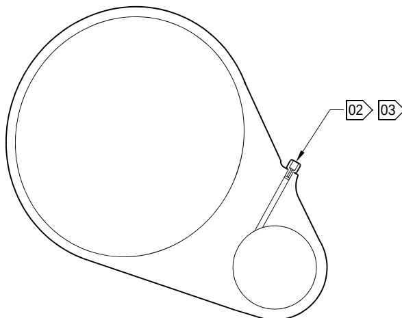
СЕЧЕНИЕ Z-Z (С СМАЗОЧНЫМ АДАПТЕРОМ)
