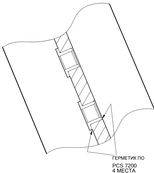
ЧАСТИЧНОЕ СЕЧЕНИЕ Z-Z С РЕМОНТНЫМИ ВТУЛКАМИ
