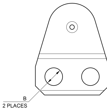
VIEW Y
