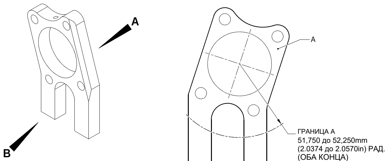
ВИД А
