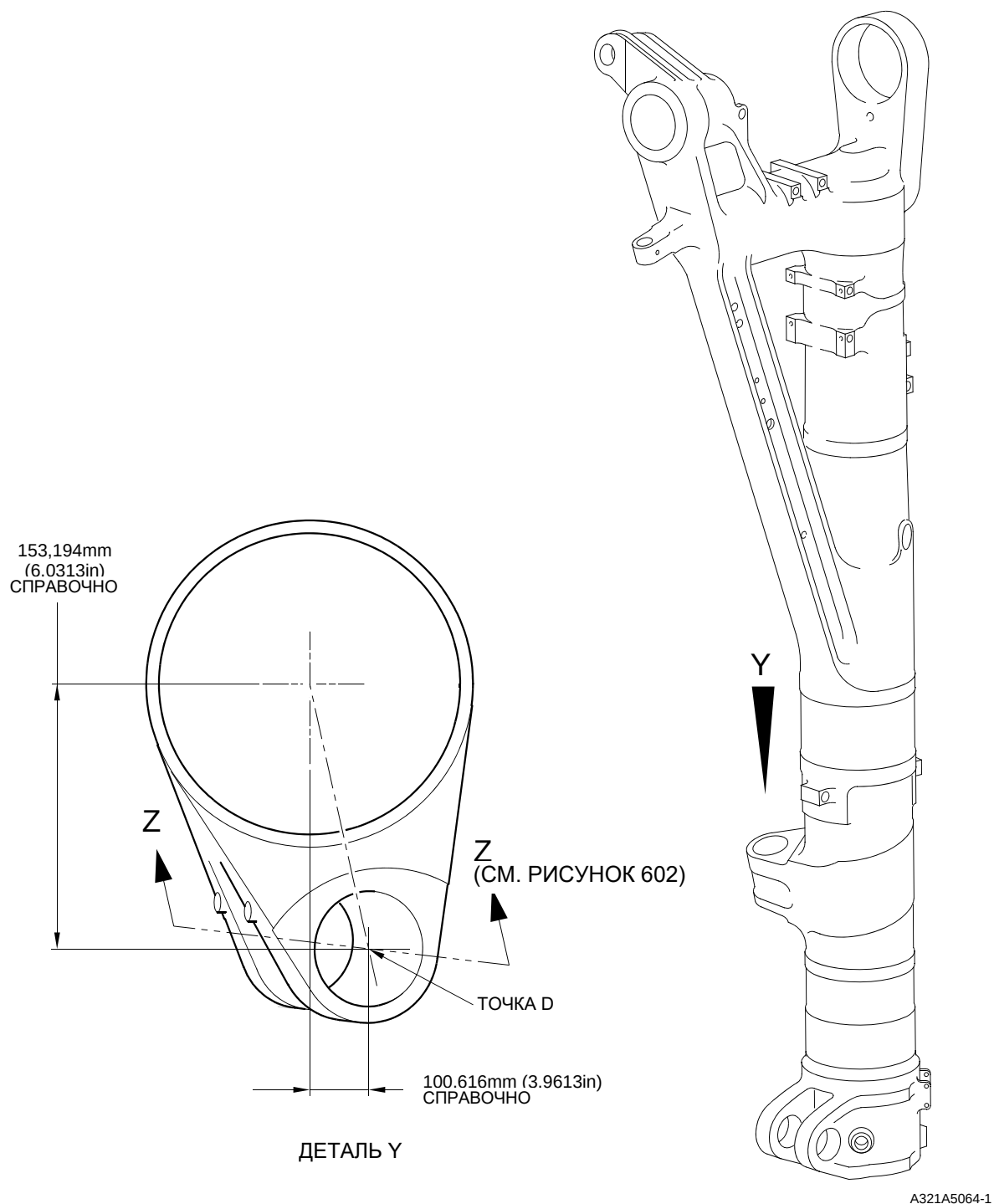
Ремонт корпуса стойки Рисунок 601
