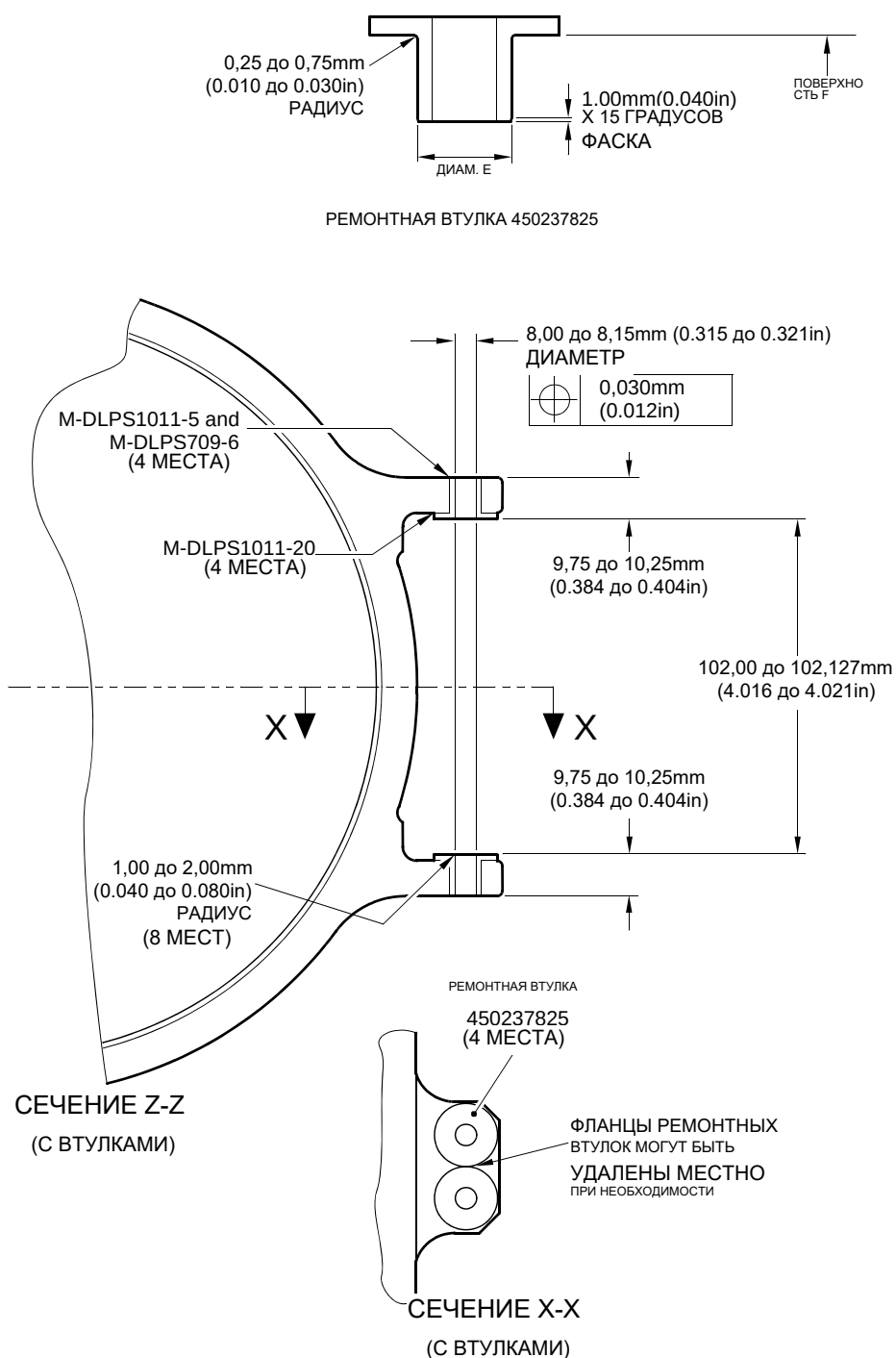
Ремонтная втулка – мехобработка и установка Рисунок 603
