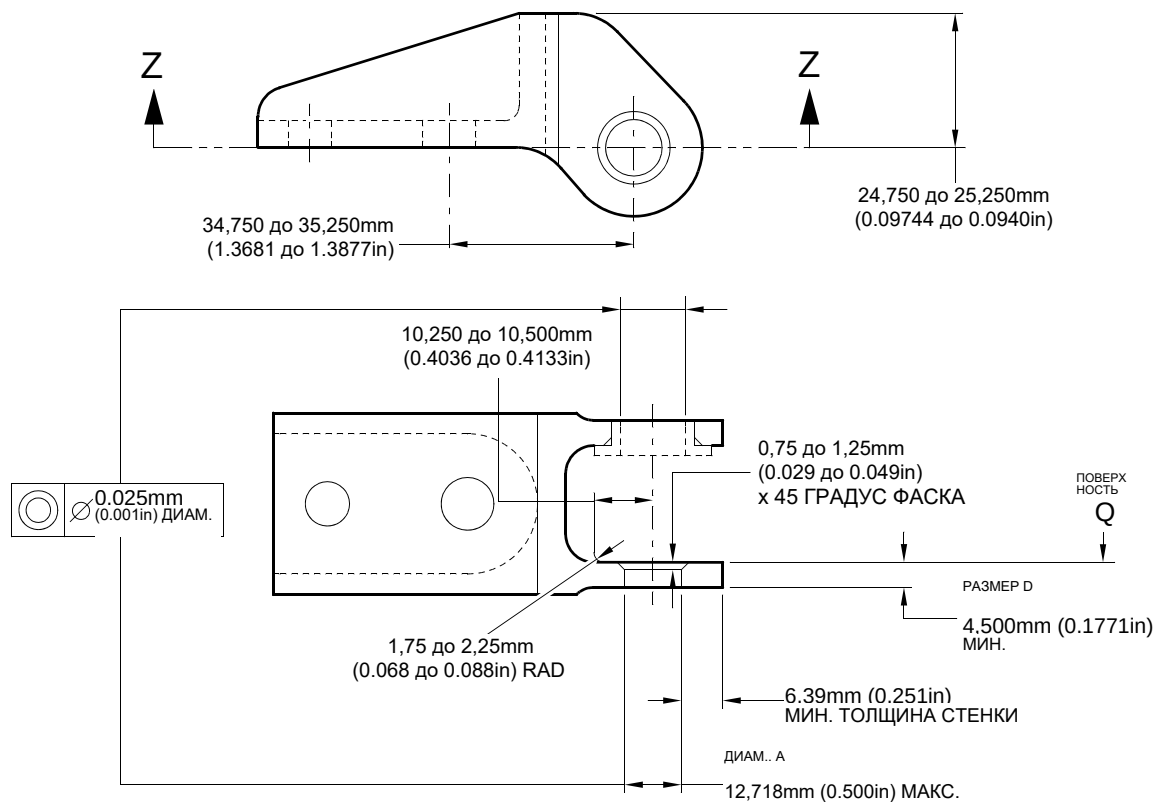
СЕЧЕНИЕ Z-Z БЕЗ ПОДШИПНИКА
