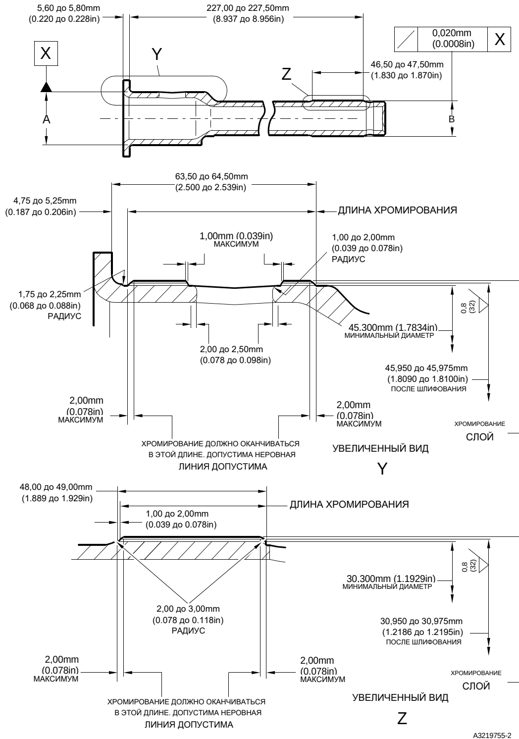
Ремонт штифта Рисунок 601
