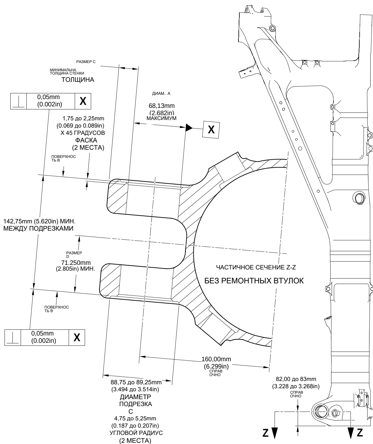
Ремонт корпуса стойки Рисунок 601
