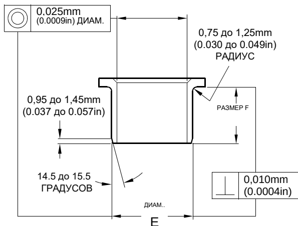
РЕМОНТНЫЙ ПОДШИПНИК 450258809
