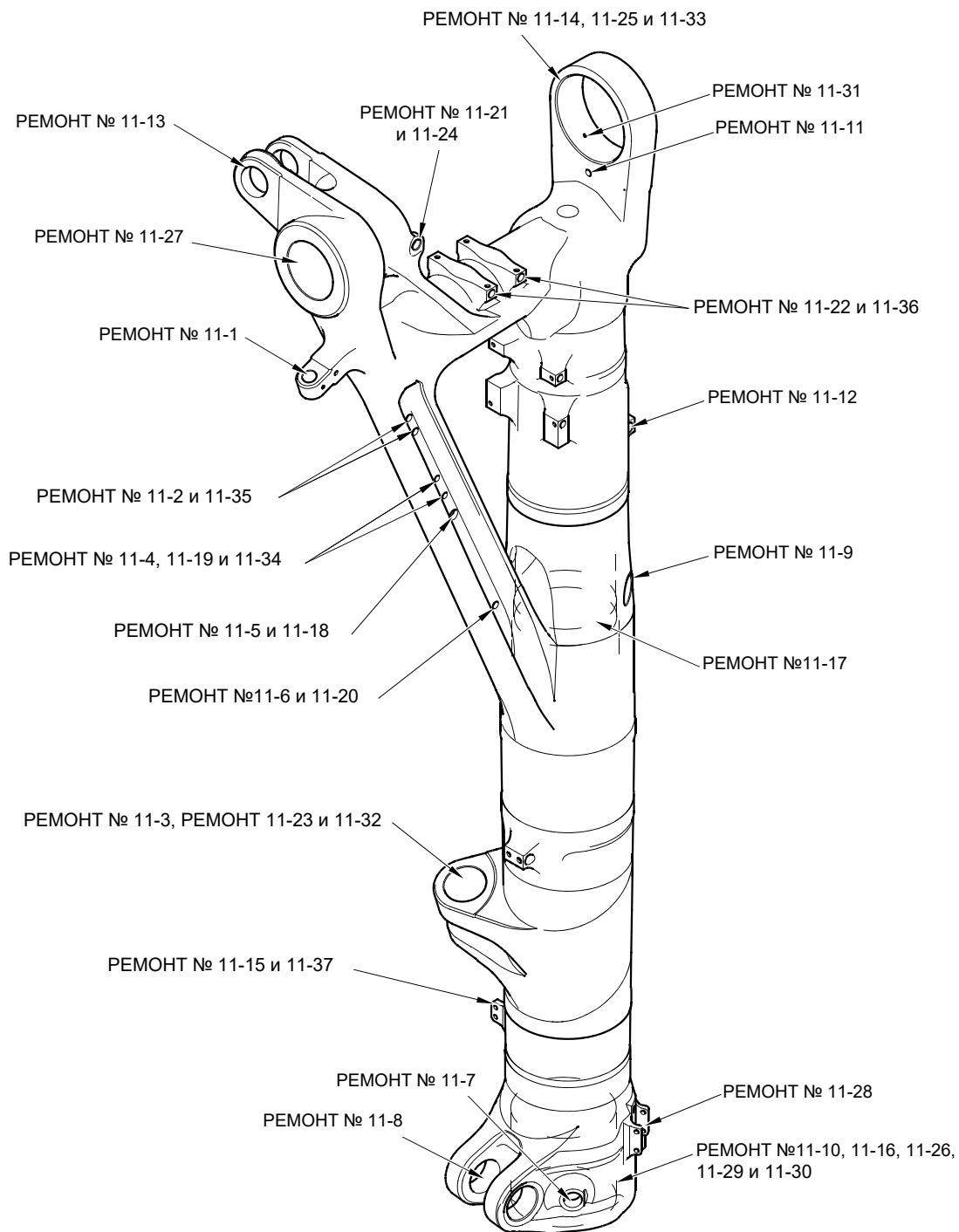
Ремонты корпуса стойки – Ключевая схема Рисунок 650
