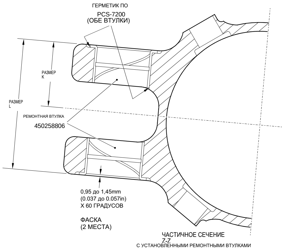
Ремонт корпуса стойки – мехобработка и установка ремонтной втулки Рисунок 602
