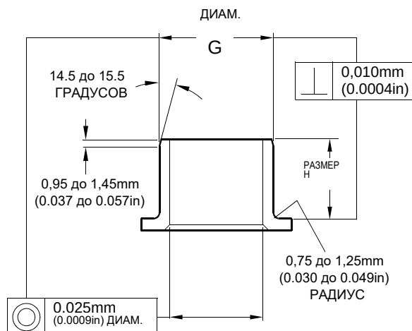
РЕМОНТНЫЙ ПОДШИПНИК 450258810
