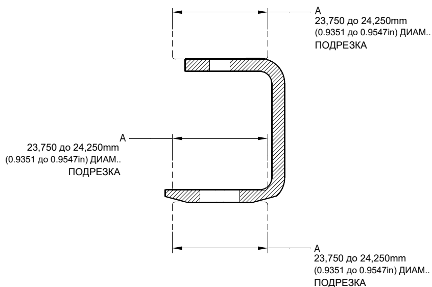
СЕЧЕНИЕ Z-Z ТИПОВО
