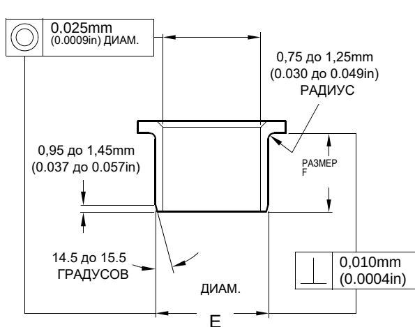
РЕМОНТНЫЙ ПОДШИПНИК 450258809
