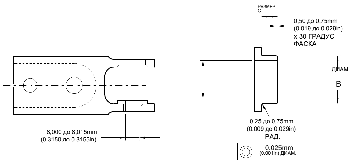
РЕМОНТНЫЙ ПОДШИПНИК – МЕХОБРАБОТКА
