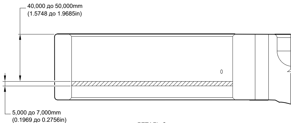
ДЕТАЛЬ С
