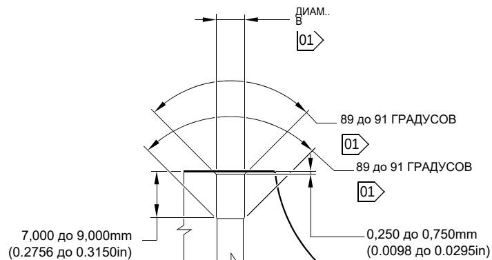
ДЕТАЛЬ В
