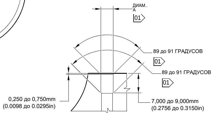
ДЕТАЛЬ С
