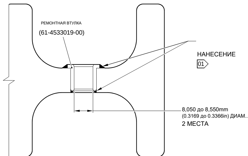
СЕЧЕНИЕ Y-Y (С ВТУЛКОЙ)
